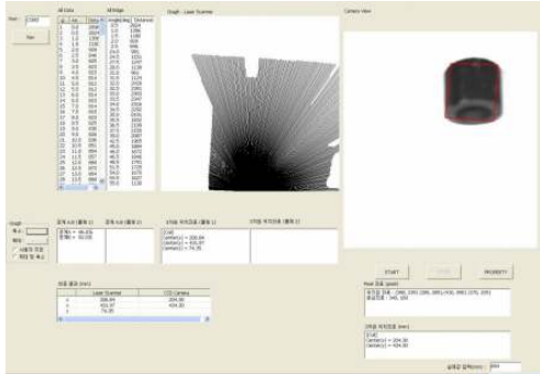
그림 11. Coil의 3차원 위치좌표 추출 결과 Fig 2. The consequence from the Slab
