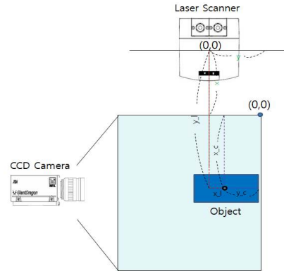
그림 9. 통합 비전 시스템에서의 위치좌표 정합
