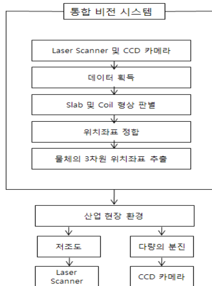
그림 4. 통합 비전 시스템 순서도 Fig 4. The flow chart of integrated vision system 그림 4는 통합 비전 시스템 순서도를 보여준다.
