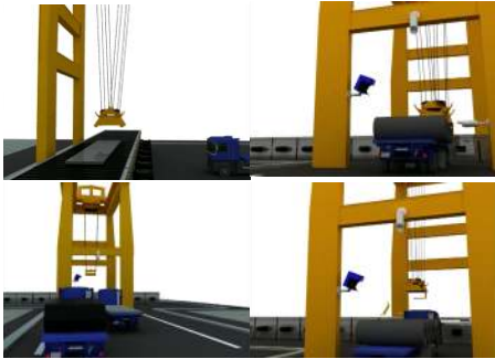
그림 1. 3DS MAX를 이용한 통합 비전 시스템의 Layout Fig 1. Layout of the integrated vision system made with 3DS MAX
