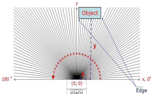
그림 5. 레이저 스캐너를 이용한 위치좌표 Fig 5. Deciding the location coordinate with laser scanner
