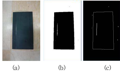
그림 6. 물체의 외곽선 추출: (a) 원본영상 (b) 이진화 영상 (c) 외곽선 추출 후 영상
