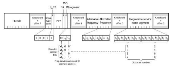
그림2. RDS Data Format of Type 0A
