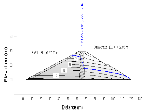
그림 3. 시간에 따른 공극수압과 수위의 변화. 그림 4. 침투류 해석에 의한 공극수압의 분포(금광)
