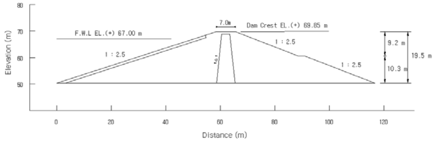
그림 1. 금광저수지의 단면
