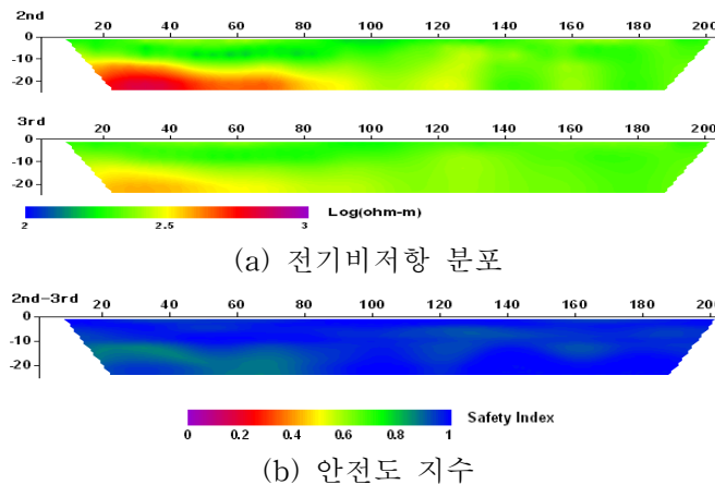
그림 8. 전기비저항과 안전도 지수 분포(금광)
