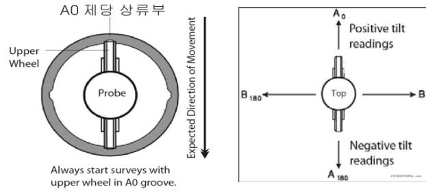
그림 5. 경사계 변위 측정축의 위치
