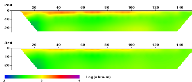
(a) 전기비저항 분포
