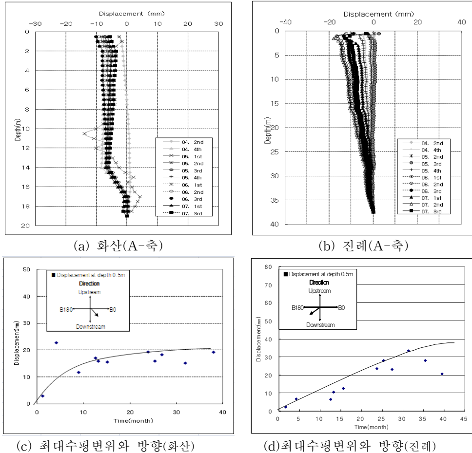
그림 7. 심도별 수평 변위량과 최대 수평변위량 및 변위방향 분포(화산, 진레)
