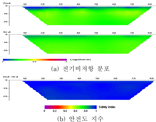
그림 9. 전기비저항과 안전도 지수 분포(경포)
