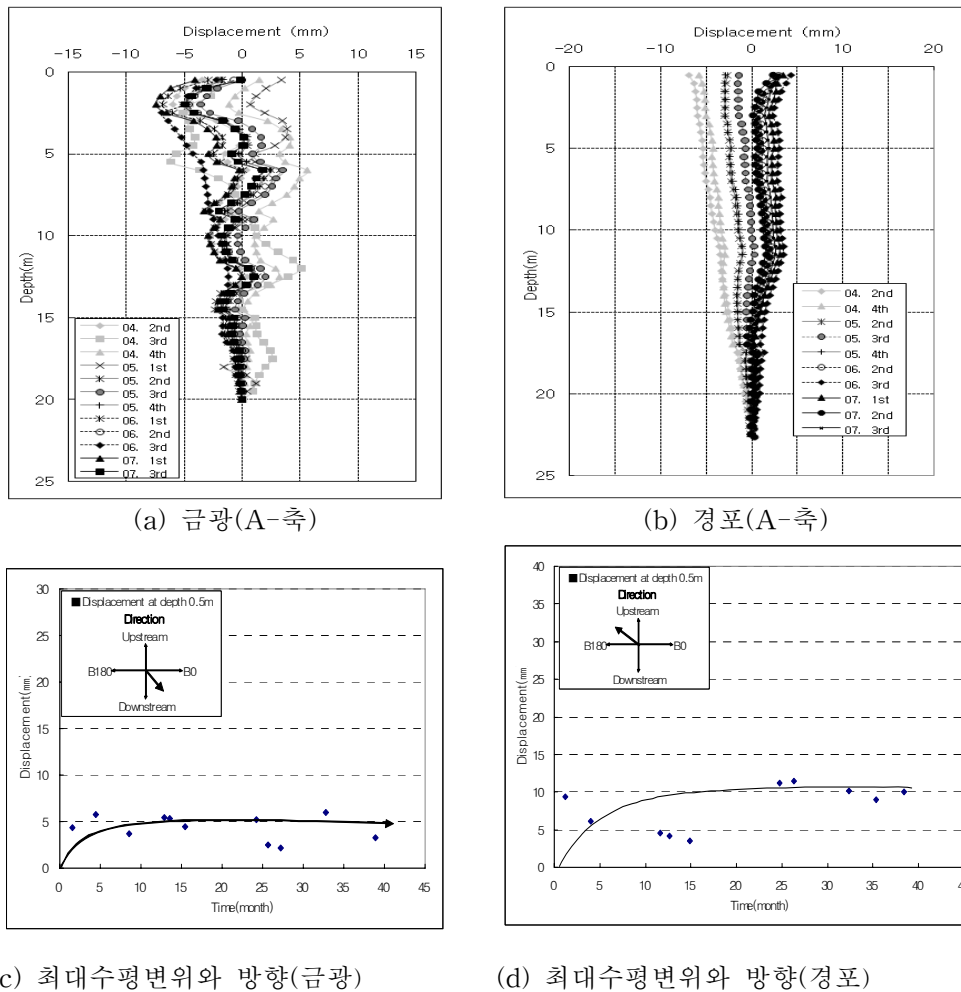
그림 6. 심도별 수평 변위량과 최대 수평변위량 및 변위방향 분포(금광, 경포)
