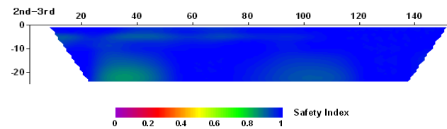
(b) 안전도 지수
