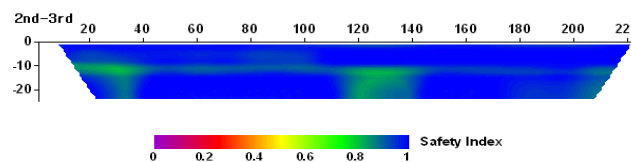
(b) 안전도 지수
