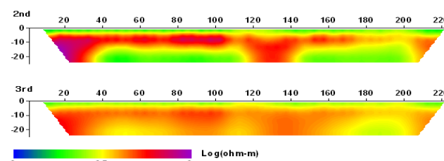
(a) 전기비저항 분포
