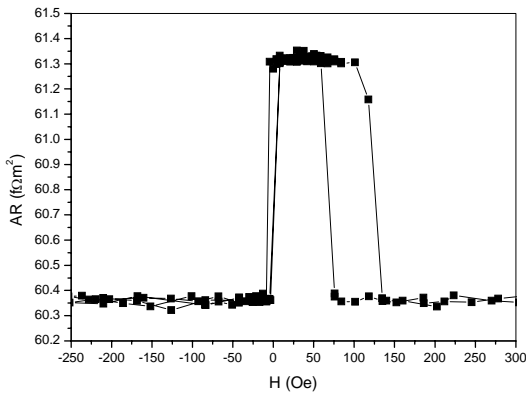
그림 1. \text{Co}_{40}\text{Fe}_{40}\text{B}_{20} 기반 교환결합바이어스 스핀밸브 소자의 자기이력 곡선. 자유층 두께 = 고정층 두께 = 20 nm
