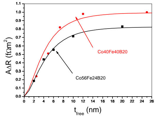
그림 2. Valet-Fert 피팅 결과 ( \text{Co}_{40}\text{Fe}_{40}\text{B}_{20} : l_{sf} \sim 4.5 nm, \beta \sim 0.3 , \text{Co}_{56}\text{Fe}_{24}\text{B}_{20} : l_{sf} \sim 4.8 nm, \beta \sim 0.26 )
