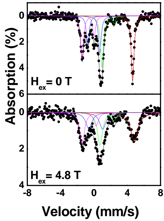
그림 1 4.2 K에서 \text{LiCo}_{0.99}\text{Fe}_{0.01}\text{PO}_4 의 Mössbauer 분광 스펙트라
