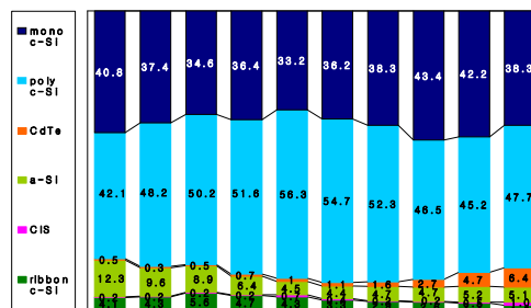
그림 5. 태양전지 기술별 점유율 추이
