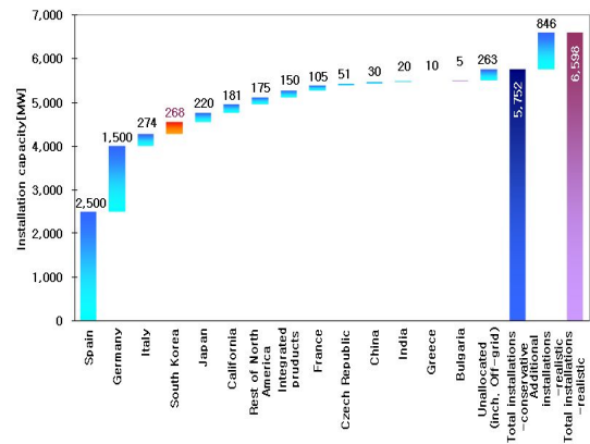
그림 9. 2008년 세계 PV설치 현황
