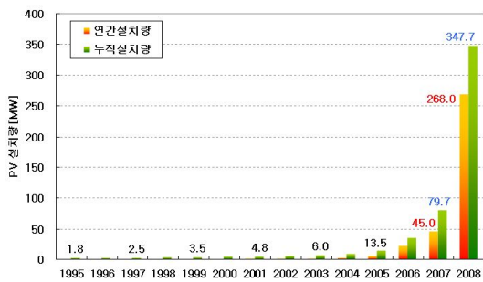
그림 8. 국내 PV 설치량 추이
