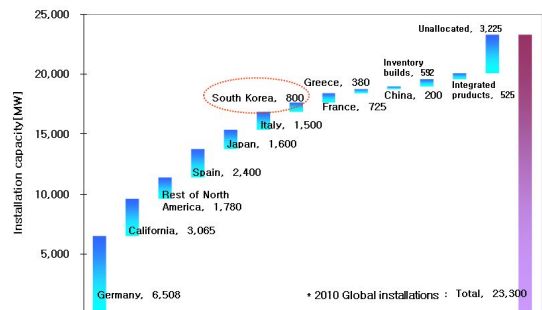
그림 10. 2010년 세계 PV설치량 예측
