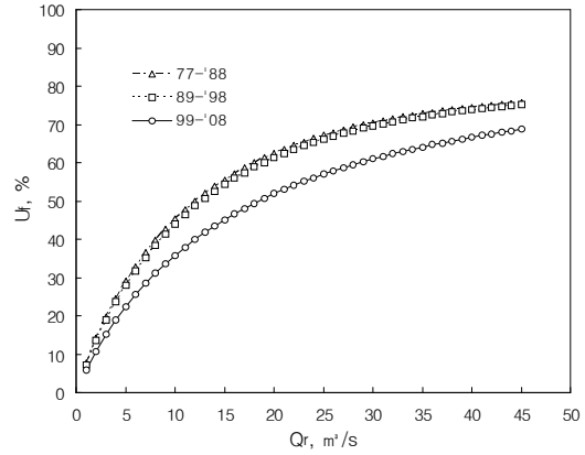
[그림 10] 기간별 이용율의 변화 예측
