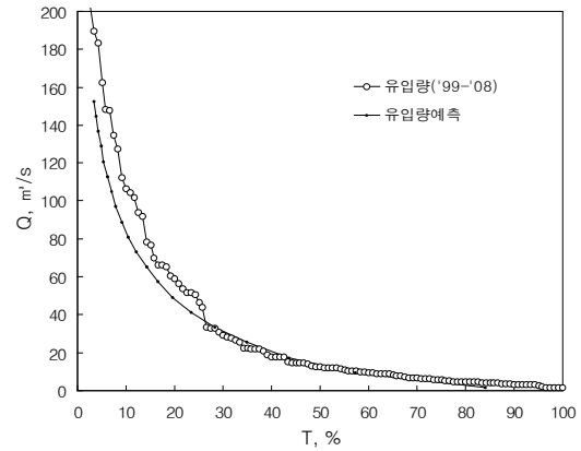
[그림 5] 안동댐 유입량 예측('99-'08)
