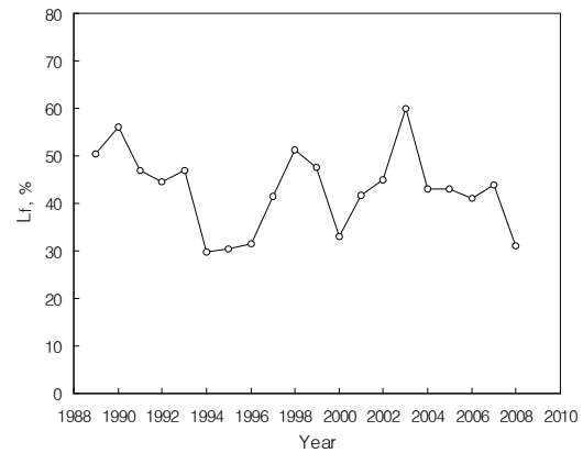
[그림 11] 연도별 연간가동율의 변화
