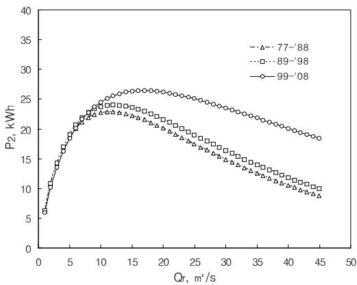
[그림 9] 기간별 정격출력량의 변화 예측
