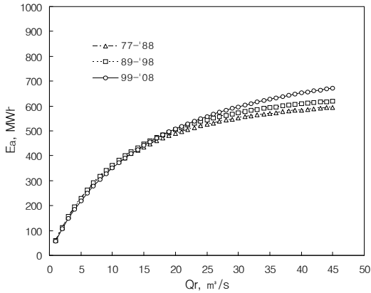
[그림 8] 기간별 연간에너지생산량의 변화 예측
