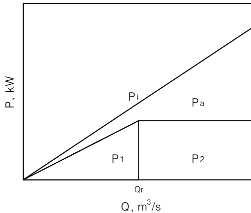
[그림 1] 소수력발전소의 출력특성
