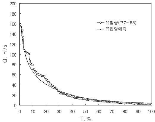
[그림 3] 안동댐 유입량 예측('77-'88)
