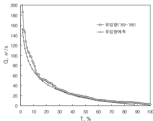
[그림 4] 안동댐 유입량 예측('89-'98)
