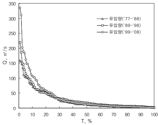
[그림 2] 안동댐 기간별 유입량
