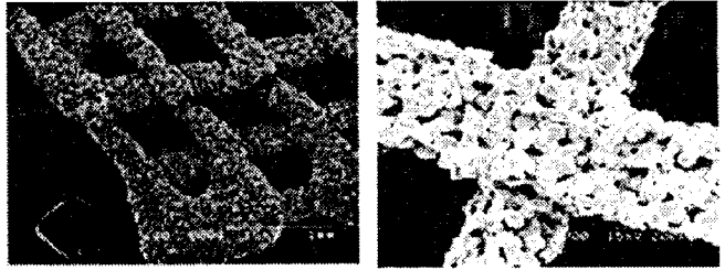
그림 3 3차원 구조의 Ti-mesh 골격 구조
