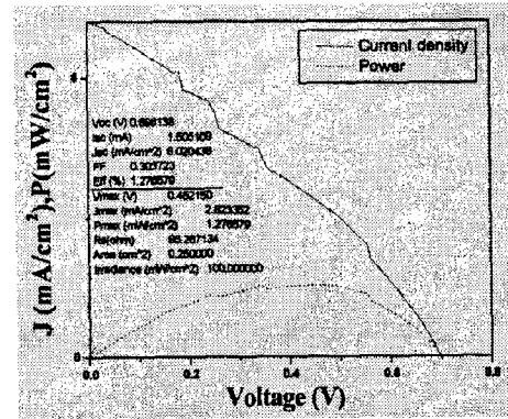
그림 5. photo-anode 층에 TiO 2 -나노입자/Ti-mesh를 사용한 DSCs의 AM1.5 하에서 광전류, 광전압 특성
