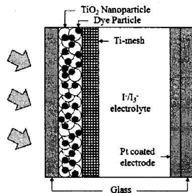
그림 1. Photo-anode 층에 TiO 2 -나노입자/Ti-mesh를 사용한 DSCs의 개략도
