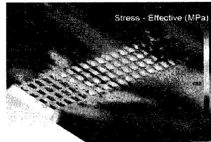
(d) After 2.85° rotation of the roll
