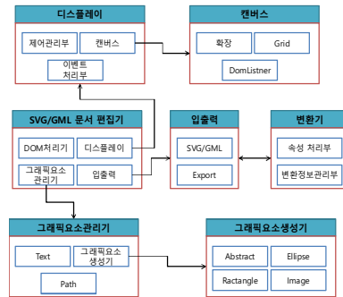
그림 1 전체 시스템 구성
