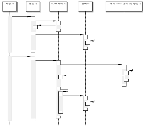
그림 4 GML 문서 편집 및 변환기 순서도
