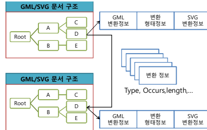
그림 3 변환 정보의 흐름도
