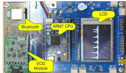
그림 7. Transferring ECG data
