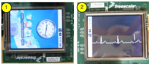
그림 9. ECG Monitoring at Android Platform
