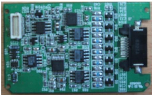
그림 1. 심전도(Electrocardiogram) 측정 모듈
