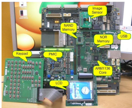
그림 5. Running Google Android on i.MX31ADS Board(ARM11)
