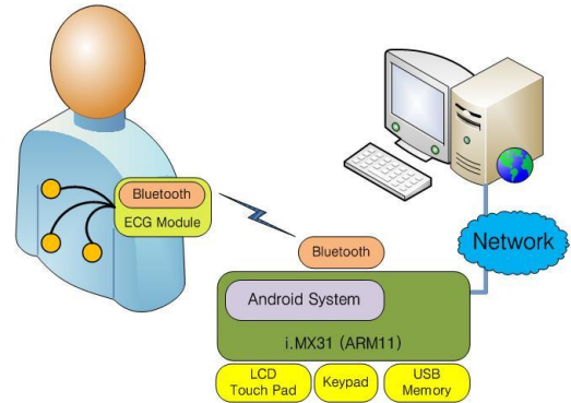
그림 6. 전체 시스템 구성도
