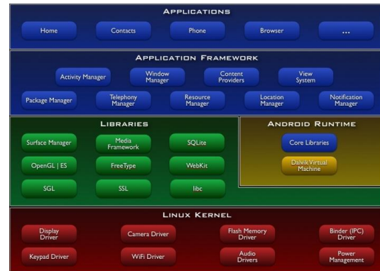
그림 3. Android Architecture
