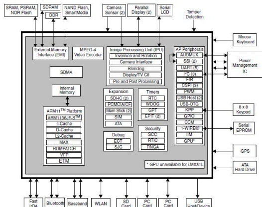
그림 4. i.MX31ADS Board Block Diagram
