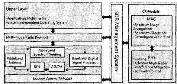
그림 4. 단말의 CR 시스템 적용 Fig. 4. The application of CR system in terminal
