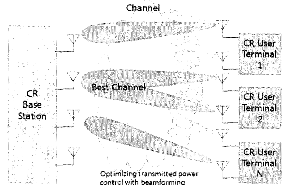
그림 3. CR 시스템에서 스마트 안테나 기술과 MIMO 기술의 적용 Fig. 3. The application of smart antenna and MIMO technique in CR system
