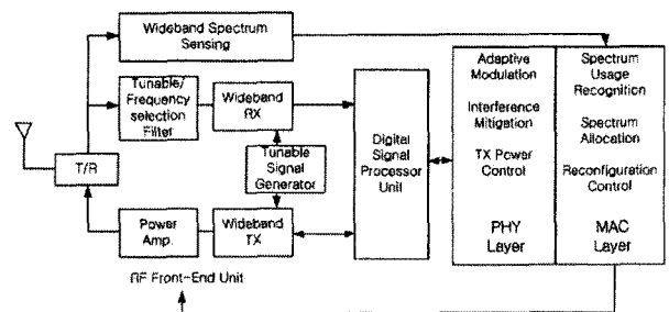
그림 2. CR 시스템 구조 Fig. 2. The structure of CR system
