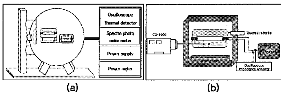
그림 2. 실험 개략도
