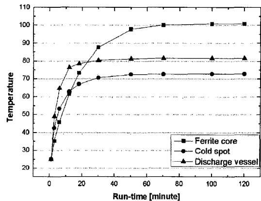
그림 4. 페라이트 코어와 방전관, 냉점의 온도변화
