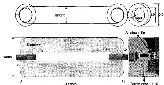
그림 1. 등근형 무전극 램프
