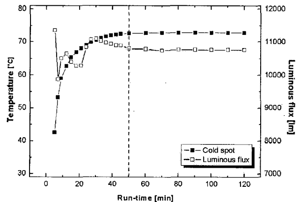
그림 5. 냉점의 온도와 광속변화 특성
