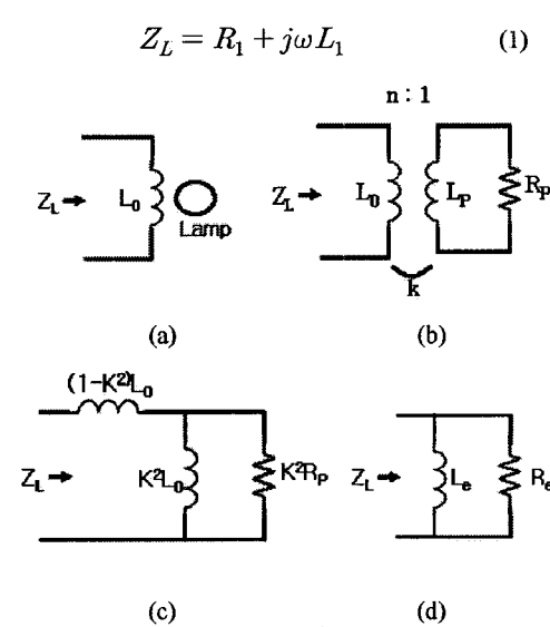
그림 3. 동근형 무전극 램프의 등가회로
