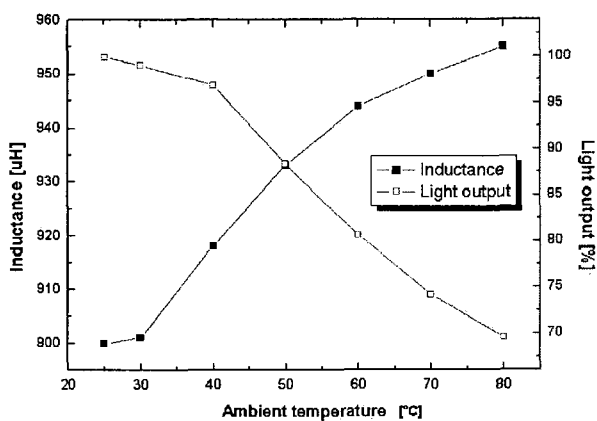
그림 7. 주변온도 증가에 따른 인덕턴스와 광출력 특성
