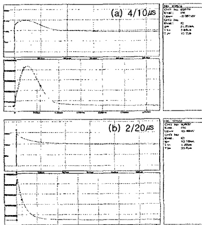
그림 2. 뇌임펄스 전류 인가에 따른 파형
