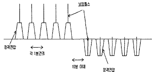
그림 1. 뇌임펄스 동작시험 패턴
