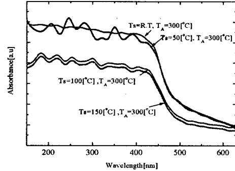
그림 3. CuGaS 2 의 흡수 스펙트럼.
