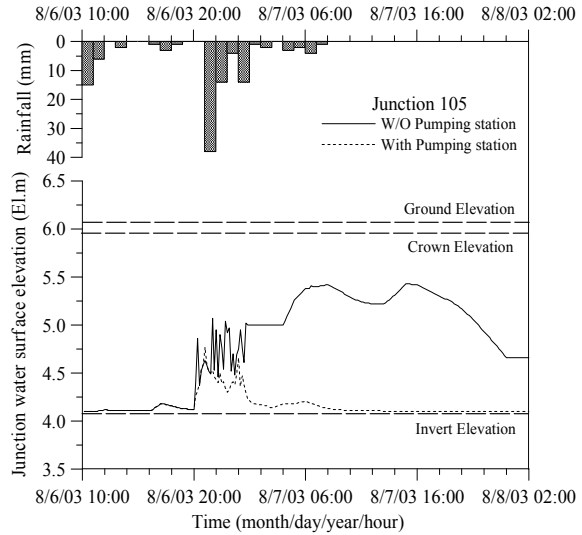
그림 9. 선유3리 배수구역 집합점 105 수위곡선
