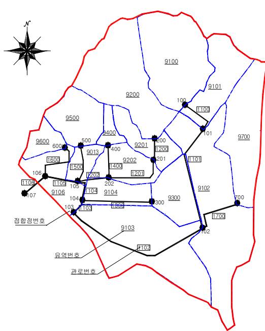
그림 1. 문산 배수펌프장 유역도
