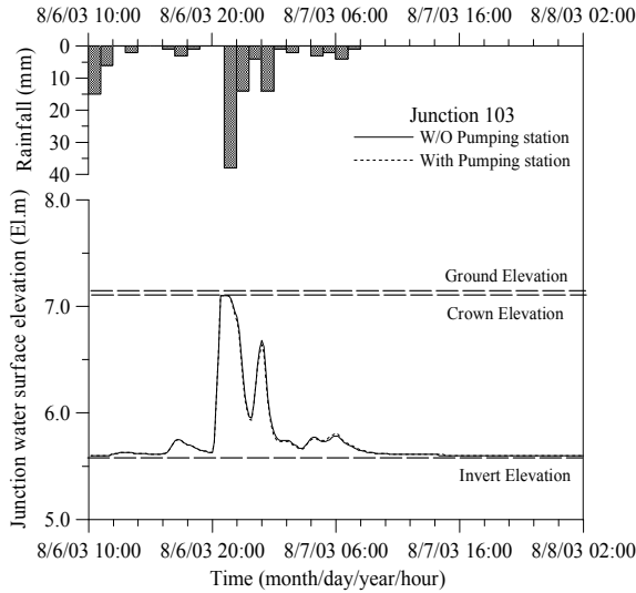
그림 8. 선유3리 배수구역 집합점 103 수위곡선
