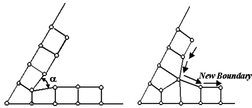
그림 8. Element reconstruction
