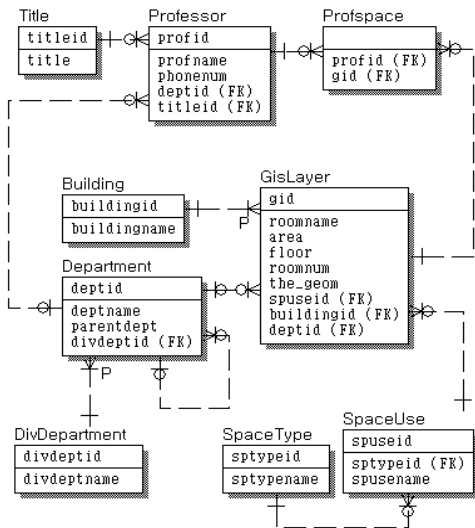
[그림 1] 시스템 E-R Diagram
