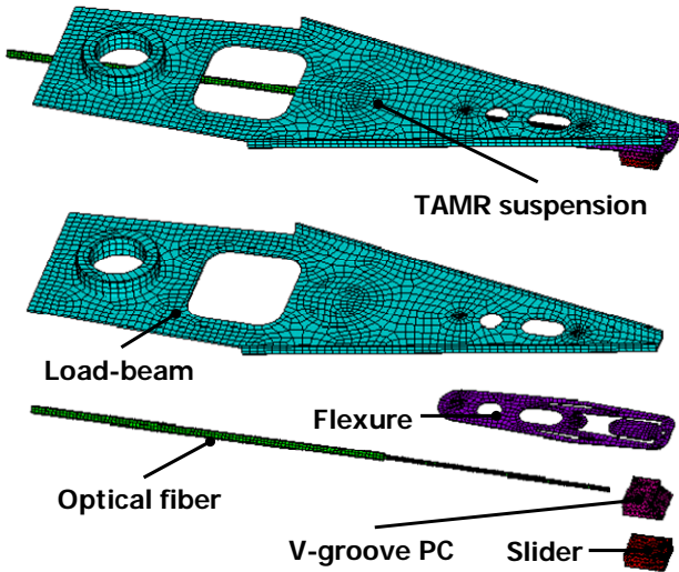
그림. 2. 열 보조 자기기록용 서스펜션
