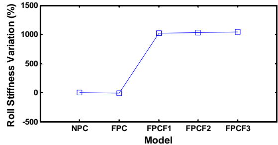
(c) 롤 강성 변화율
