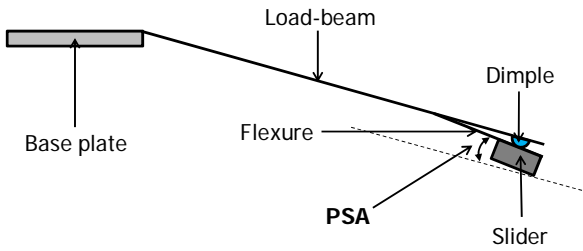
그림. 1. 서스펜션의 PSA
