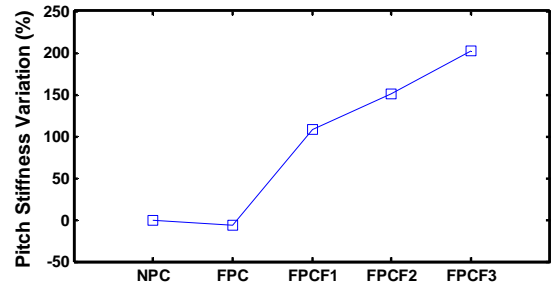
(b) 피치 강성 변화율
