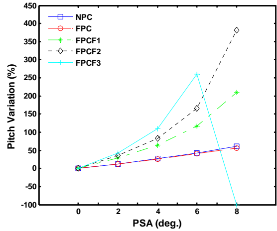
(b) 다양한 PSA 에 대한 피치의 변화율
