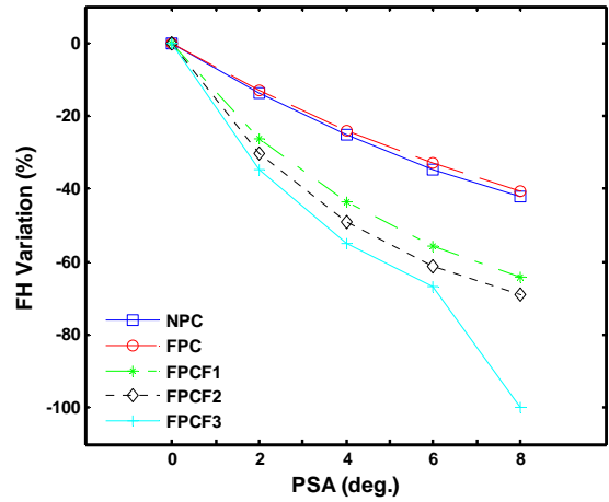
(a) 다양한 PSA 에 대한 부상 높이의 변화율
