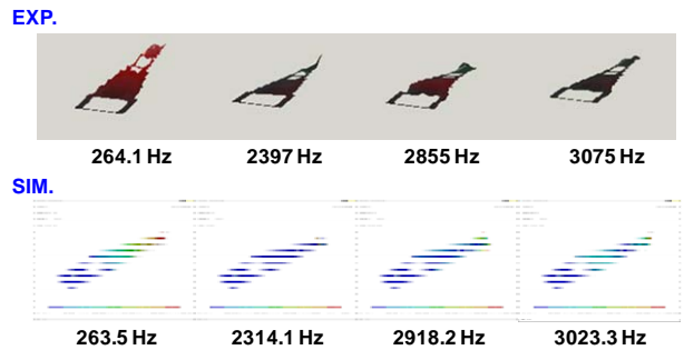
그림. 4. 모드해석 결과
