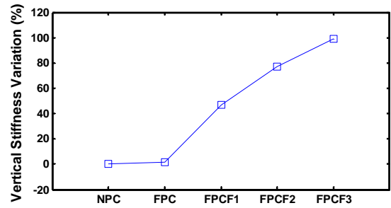
(a) 수직 강성 변화율
