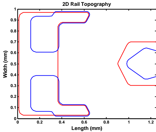
그림. 7. 슬라이더 레일 형상
