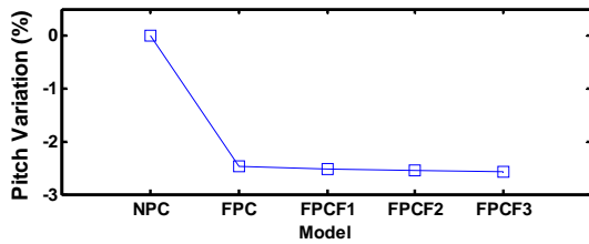
그림. 8. 각 모델에 대한 부상특성
