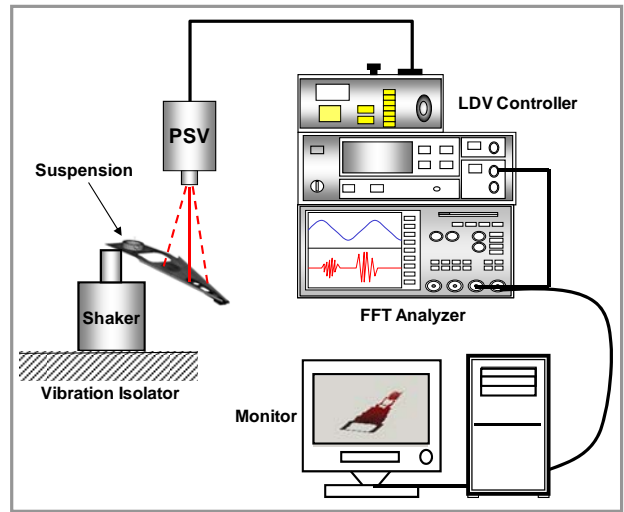
그림. 3. 모드해석 실험
