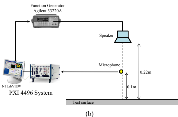
Fig 3. (a) 실험에 사용된 송, 수신자 및 측정대상 사진 (b) 실험장치 개략도
