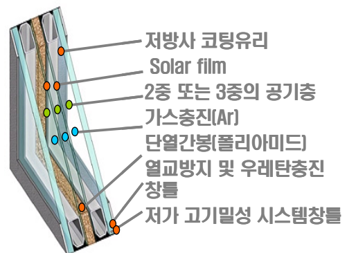
그림 1. 단열창호 슈퍼윈도우의 개념도
