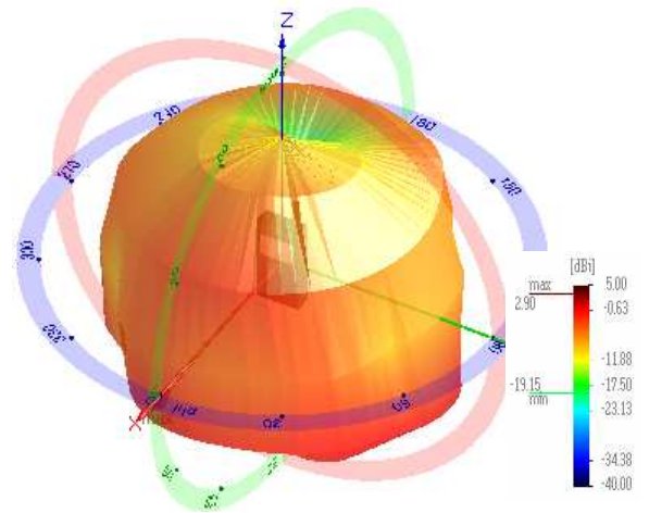
[그림 9] DCS/PCS 대역에서의 3D 방사패턴
