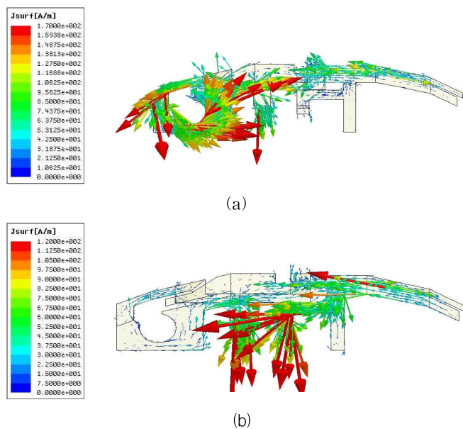
[그림 2] 대역별 전류밀도 시뮬레이션 결과: (a) GSM, (b) DCS/PCS
