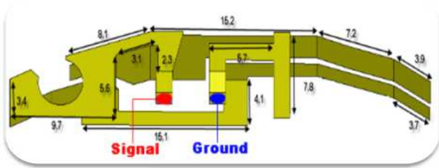
[그림 1] 제안된 안테나
