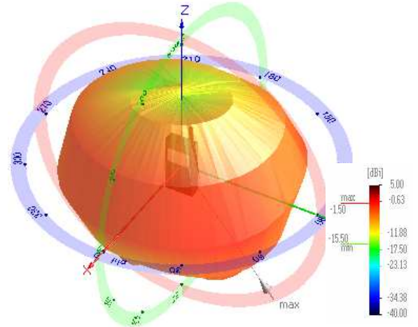
[그림 8] GSM 대역에서의 3D 방사패턴
