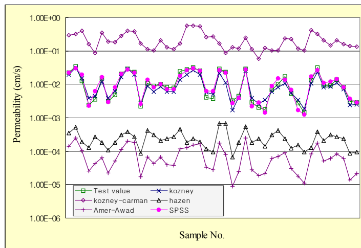
그림 7. 직접투수시험, 경험식, 그리고 투수계수산정모델에 의한 투수계수의 관계
