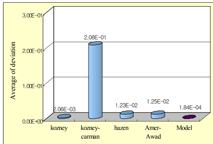
그림 8. 직접투수시험을 기준으로 각각의 방법에 의한 평균 투수계수의 편차 비교
