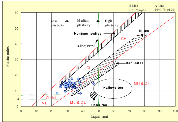
그림 2. 소성도로 나타낸 연구지역 토층시료의 액성한계 및 소성한계 시험결과
