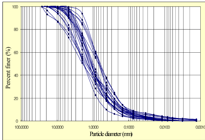
그림 3. 연구지역 대표적 토층시료의 입도분포도
