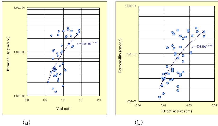
그림 4. 연구지역 토층시료의 간극비, 유효경 및 투수계수간의 관계: (a), 간극비와 투수계수; (b), 유효경과 투수계수
