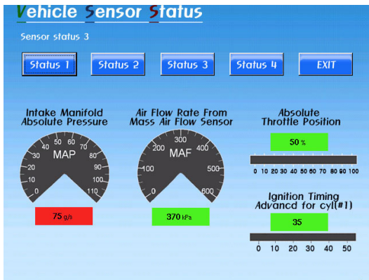
그림 12. 센서 상태 3
