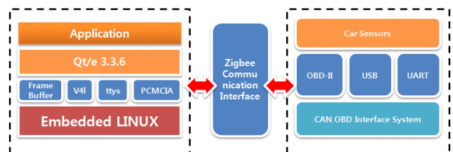
그림 7. 임베디드 소프트웨어 플랫폼
