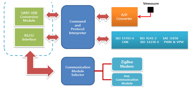
그림 6. 자동차 센서 정보 전송을 위한 ZigBee 통신 인터페이스 모듈
