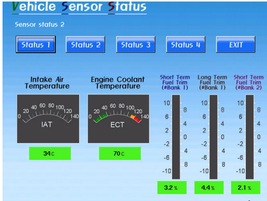
그림 11. 센서 상태 2
