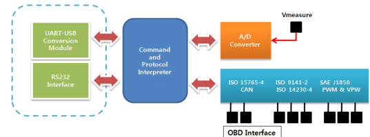
그림 3. CAN 통신 차량 센서 정보 전송장치 블록도
