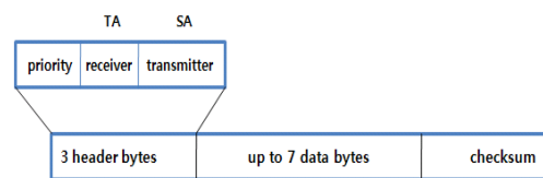
그림 4. An OBD Message
