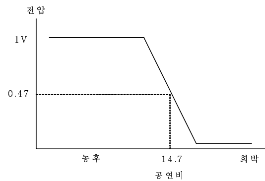
그림 14. O2센서 산소 농도차에 의한 출력전압의 변화
