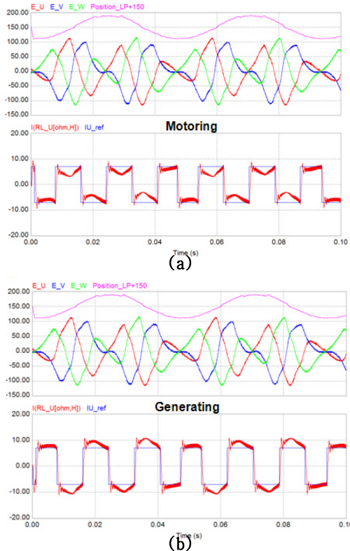
Fig. 10 동일 위치의 전동/발전모드시 U상 전류 (a) 전동모드, (b) 발전모드
