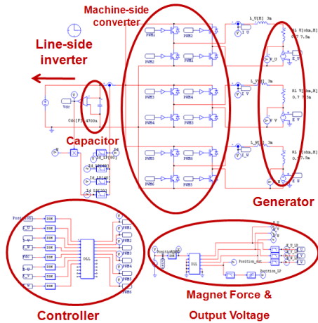
Fig. 9 시뮬레이션 모델
