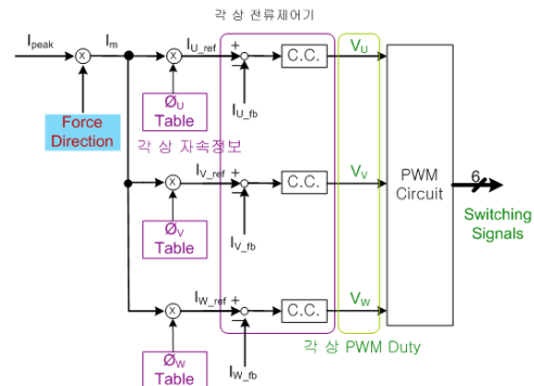
Fig. 7 전동모드시 전류 제어
