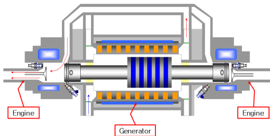
Fig. 2 선형 발전기 구조
