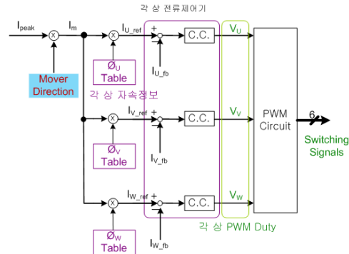
Fig. 8 발전모드시 전류 제어
