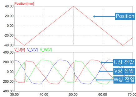
Fig. 6 등속운동 시 출력전압 [30Hz]
