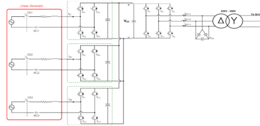
Fig. 3 선형발전기용 PCS 구조
