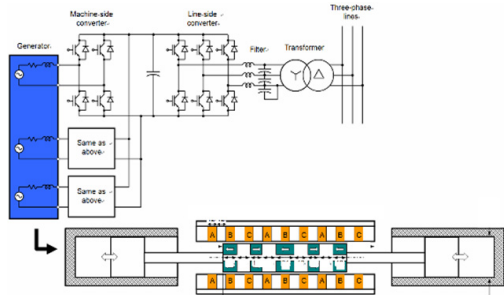
Fig. 1 선형 동력/발전 시스템 구성도
