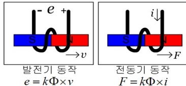
Fig. 5 발전기 및 전동기 동작원리
