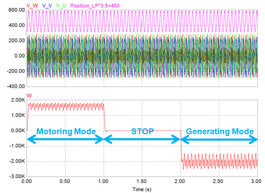
Fig. 11 전동모드→PCS정지→발전모드 시퀀스 test
