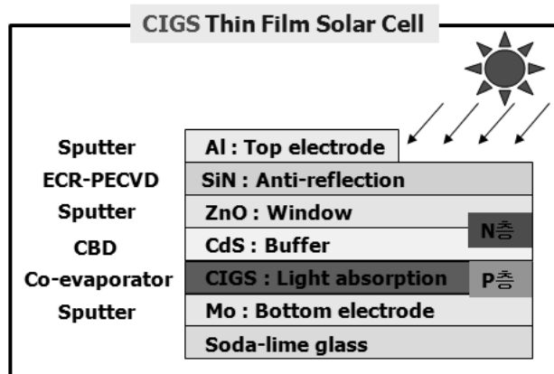
CIGS TFSC 구조와 제조용 장비
