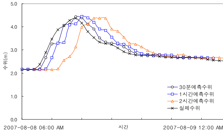
그림 2. U-FFS에 의한 예측수위 및 실측수위 비교 그래프
