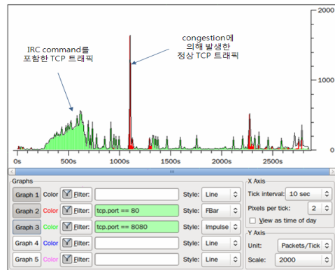
(그림 4) 포트별 PPS 분포
