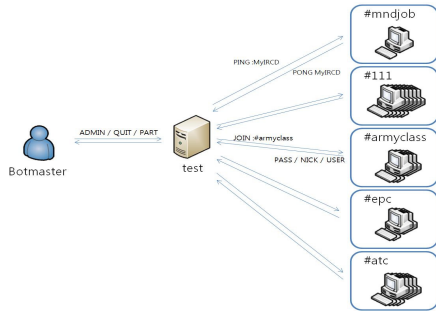
(그림 6) 트래픽 분석을 통해 밝혀진 봇넷의 구조
