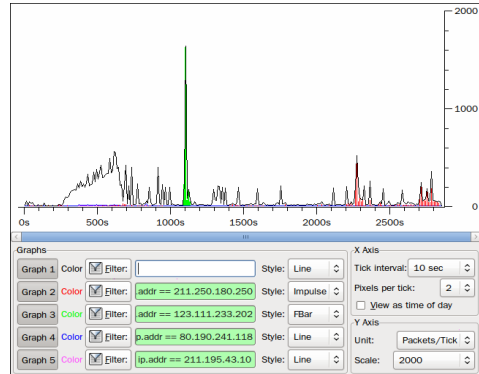
(그림 3) 빈출 IP 에 따른 PPS 분포
