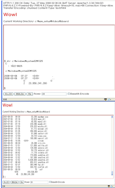
(그림 5) 봇마스터의 호스트 폴더 검색 행위
