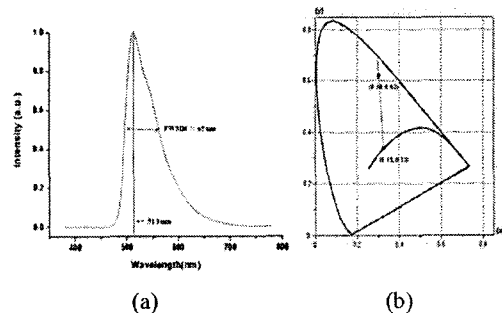
그림 3. 전기발광 스펙트럼(a)과 CIE 색 좌표(b).
