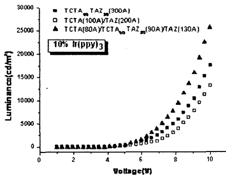
그림 1. 휘도-전압 특성.
