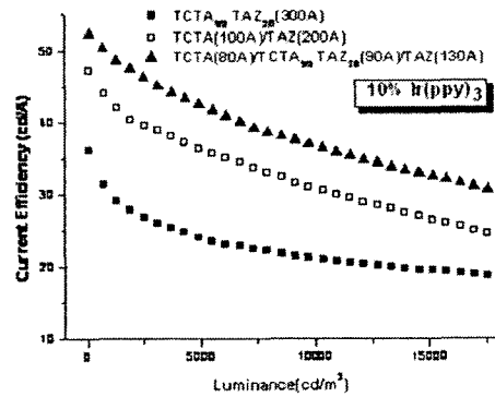
그림 2. 전류효율-휘도 특성.
