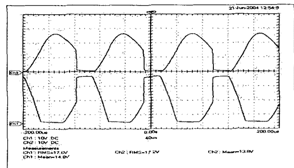
그림 7. Tp1에서의 전압파형
