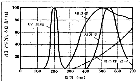
그림 3. UV tron의 스펙트럼 특성
