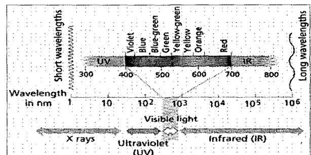
그림 1. 태양광의 스펙트럼 분포
