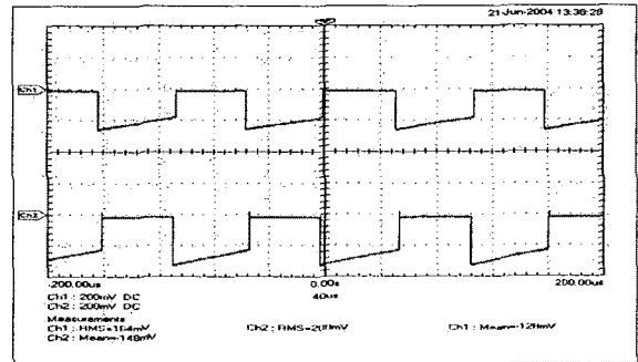
그림 6. PWM 제어 파형
