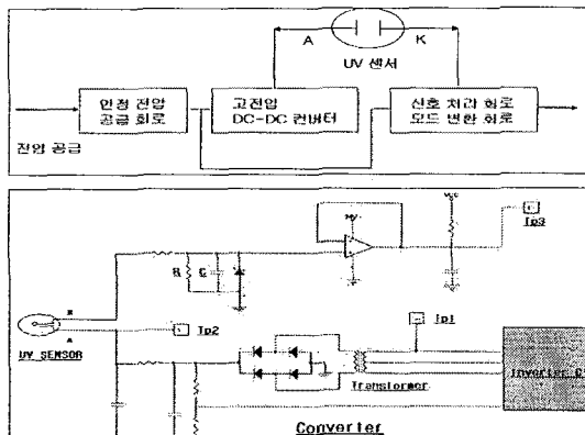
그림 5. 회로 블록도와 실험 회로
