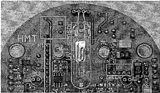
그림 10. UV센서 응용 회로설계 PCB
