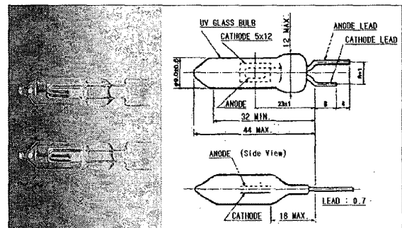
그림 4. 제품화된 광전관
