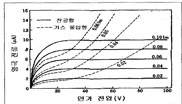
그림 2. 전압에 따른 양극 전류와의 관계
