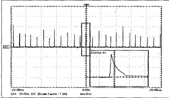
그림 9. UV tron의 출력 전압 파형
