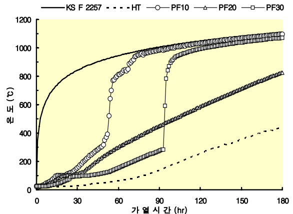
그림 1 ECC 피복부 두께에 따른 온도이력곡선
