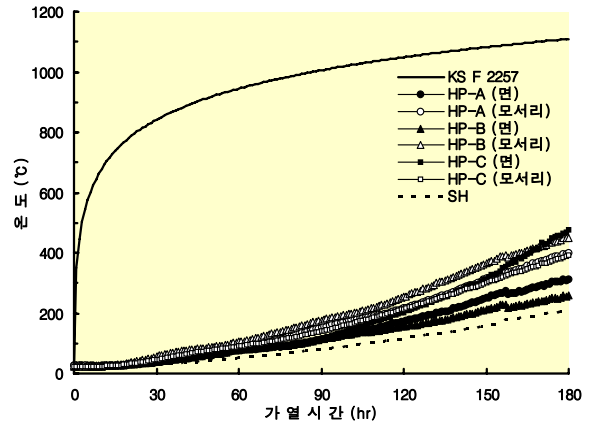
그림 2 내화충전재 종류에 따른 온도이력곡선
