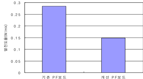
그림 3. 열전도율 시험 결과
