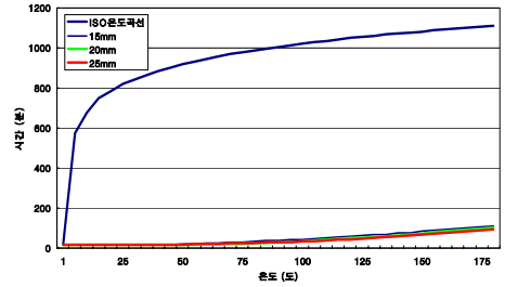
그림 6 3시간 내화시험 결과
