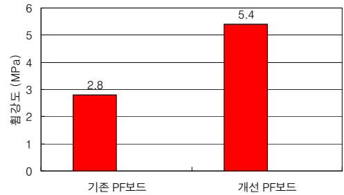
그림 1. 휨강도 시험 결과
