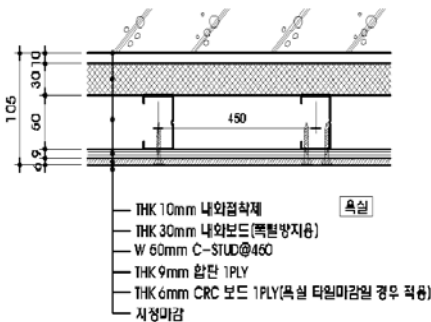
그림 7 습식 PFB 공법 상세설계도
