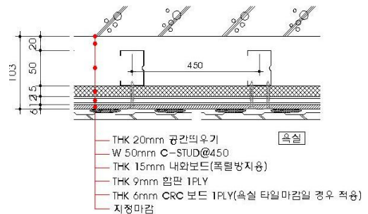
그림 8 건식 PFB 공법 상세설계도
