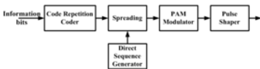
▶▶ 그림 1. The Transmission diagram of DS-PAM-UWB
