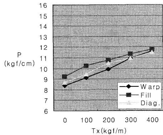
그림6 막장력값(Tx)과 Push-Pull게이지값(P) 곡선 (Ty=400 kg/m, Tip=75mm의 경우)
