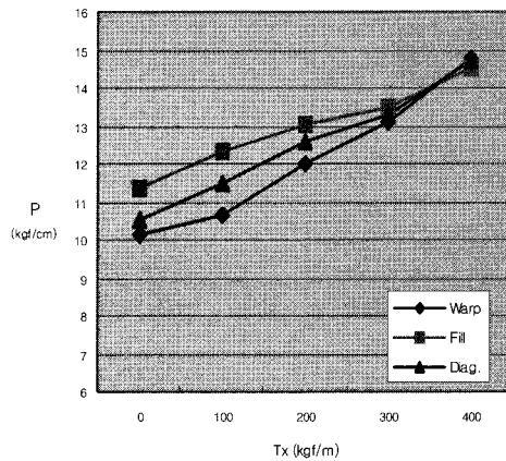
그림11 막장력값(Tx)과 Push-Pull게이지값(P) 곡선 (Ty=400 kg/m, TL=100mm의 경우)
