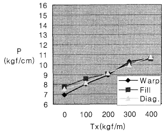
그림5 막장력값(Tx)과 Push-Pull게이지값(P) 곡선 (Ty=200 kg/m, Tip=75mm의 경우)
