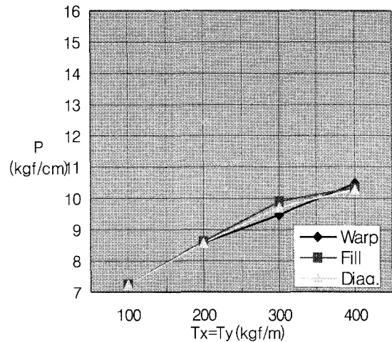
그림13 Tx=Ty시의 Push-Pull게이지값(P) 곡선 (TL=50mm 사용)
