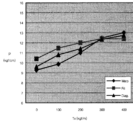
그림10 막장력값(Tx)과 Push-Pull게이지값(P) 곡선 (Ty=300 kg/m, TL=100mm의 경우)
