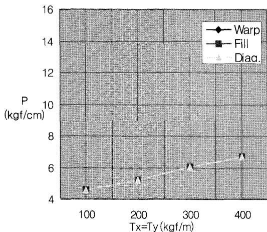
그림12 Tx=Ty인 경우 Push-Pull게이지값(P) (원형 Tip 사용)
