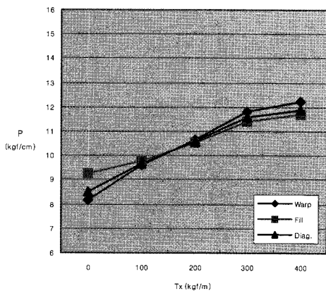
그림9 막장력값(Tx)과 Push-Pull게이지값(P) 곡선 (Ty=200 kg/m, TL=100mm의 경우)
