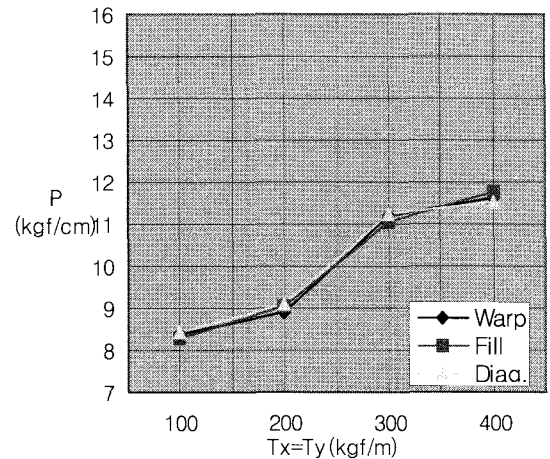
그림14 Tx=Ty시의 Push-Pull게이지값(P) 곡선 (TL=75mm 사용)
