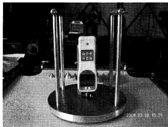
사진1 휴대용 막장력 측정기(PTMM) 형상
