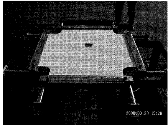
사진3 2축 장력시험기 실물 사진
