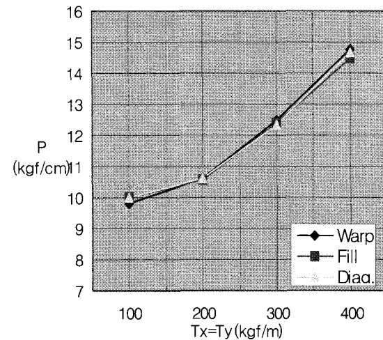
그림15 Tx=Ty시의 Push-Pull게이지값(P) 곡선 (TL=100mm 사용)
