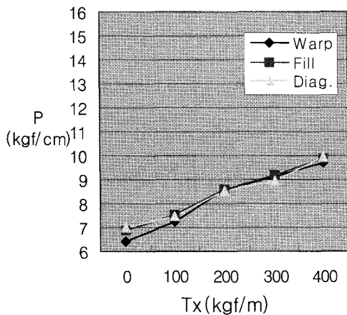
그림3 막장력값(Tx)과 Push-Pull게이지값(P) 곡선 (Ty=200 kg/m, Tip=50mm의 경우)
