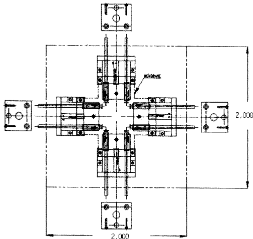
그림2 2축 장력시험기 평면도
