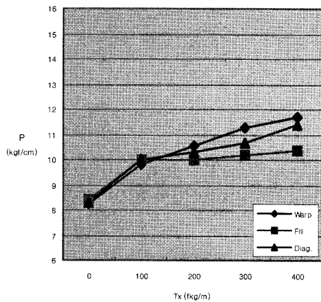
그림8 막장력값(Tx)과 Push-Pull게이지값(P) 곡선 (Ty=100 kg/m, TL=100mm의 경우)
