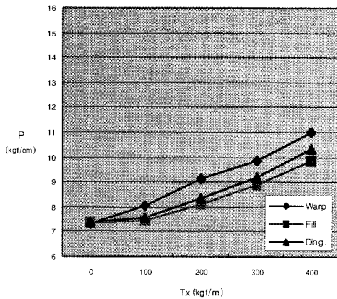
그림7 막장력값(Tx)과 Push-Pull게이지값(P) 곡선 (Ty=0 kg/m, TL=100mm의 경우)
