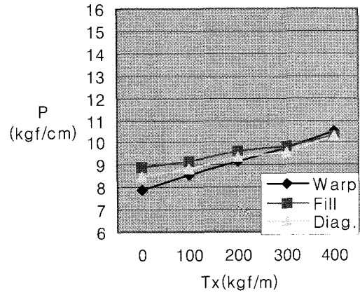
그림4 막장력값(Tx)과 Push-Pull게이지값(P) 곡선 (Ty=400 kg/m, Tip=50mm의 경우)
