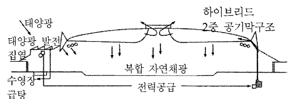
〈그림 3〉 하이브리드 태양광 시스템 개념도
