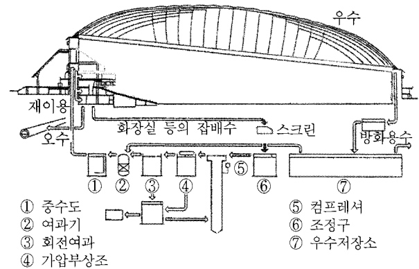
〈그림 2〉 도쿄돔의 우수·중수이용 계통도
