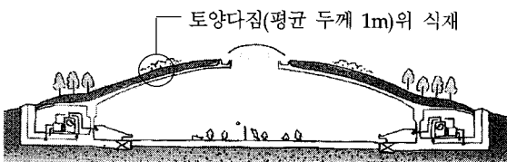
〈그림 1〉 오사카 중앙체육관 단면
