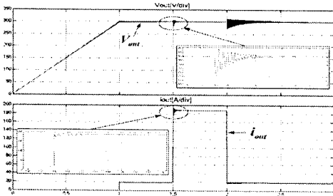
그림 8 PI제어기만 적용한 경우 Fig. 8 PI controller without load current feedforward
