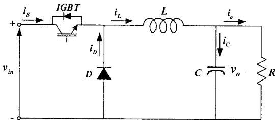
그림 2 강압초퍼 Fig. 2 Step-down chopper
