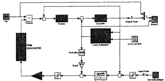
그림 7 강압초퍼의 simulink 블록도 Fig. 7 Simulink block diagram of Step-down chopper
