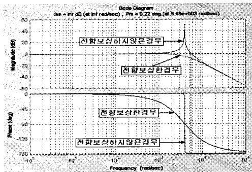
그림 6 부하전류 전향보상기에 따른 시스템의 주파수 응답 Fig. 6 The frequency response of system based on load current feedforward
