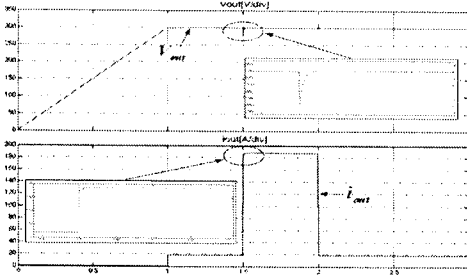
그림 9 부하전류 전향보상기를 적용한 경우 Fig. 9 PI controller with load current feedforward
