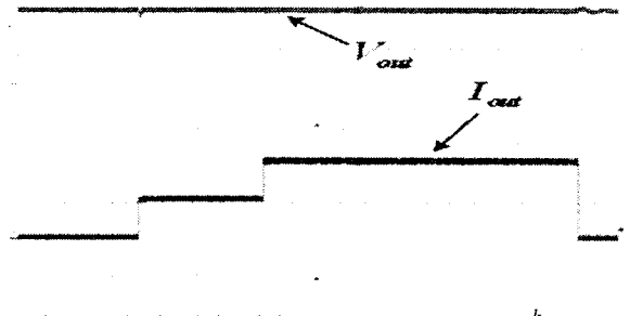
그림 12 부하전류 전향보상기를 적용한 경우 출력파형( k_f=0.5 ) Fig. 12 Output waveforms of step-down chopper with load current feed-forward compensator( k_f=0.5 ) (3. 50(V/Div), 4. 10(A/Div) Time Div 200(msec))
