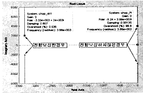
그림 5 부하전류 전향보상기에 따른 시스템의 근궤적 Fig. 5 The Root locus of system based on load current feedforward
