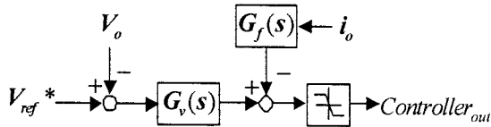
그림 1 전향보상기를 포함한 시스템 제어블록도 Fig. 1 Control block diagram including feedforward compensator
