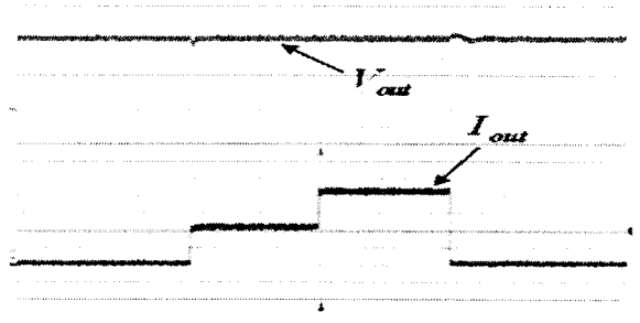
그림 11 PI제어기만 적용한 경우 강압쇼퍼의 출력파형 Fig. 11 Output waveforms of a step-down chopper with PI controller (3. 50(V/Div), 4. 10(A/Div) Time Div 200(msec))
