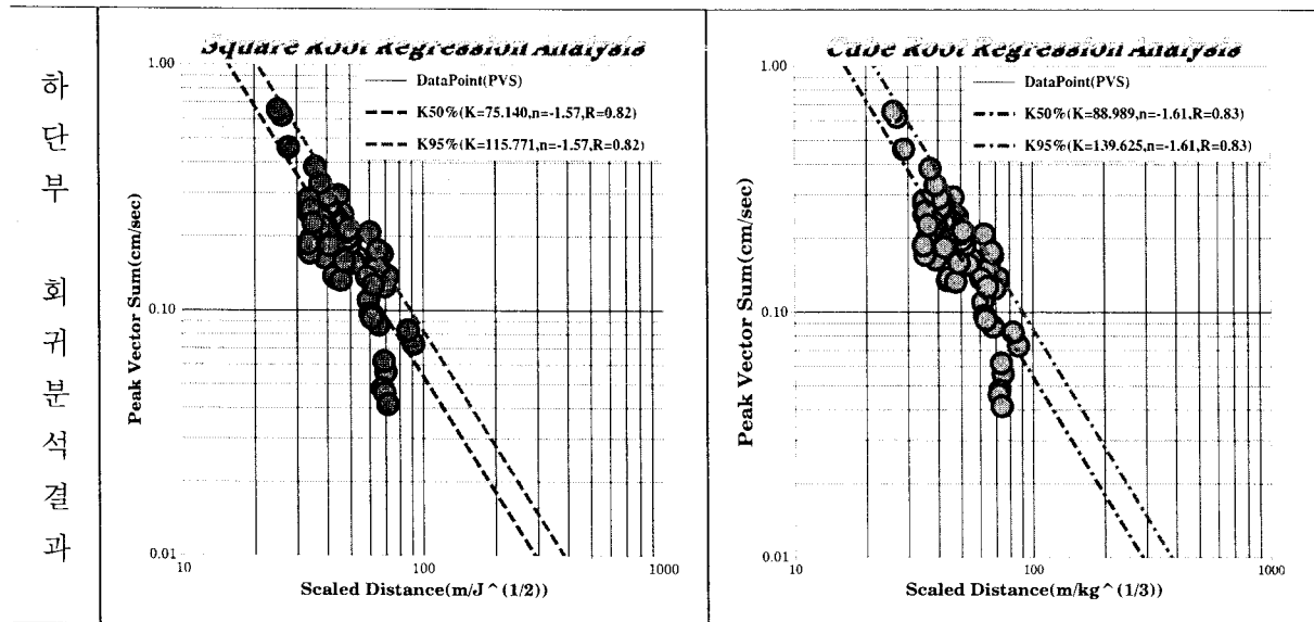
그림 3.1(b) 하부반단면 회귀분석결과
