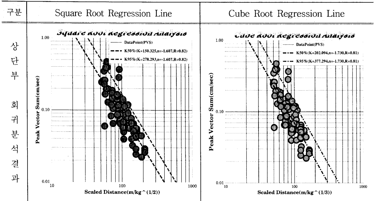
그림 3.1(a) 상부반단면 회귀분석결과
