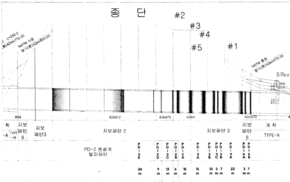
그림 3.1(a) 상단부터널 발파구간별 적용발파패턴 구분(단면도)
