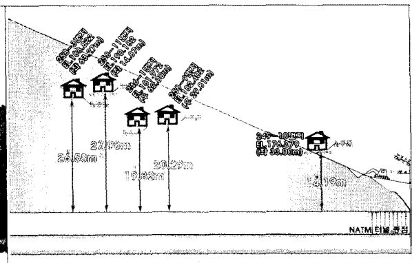
그림 2.2 터널과 보안물건과의 이격거리
