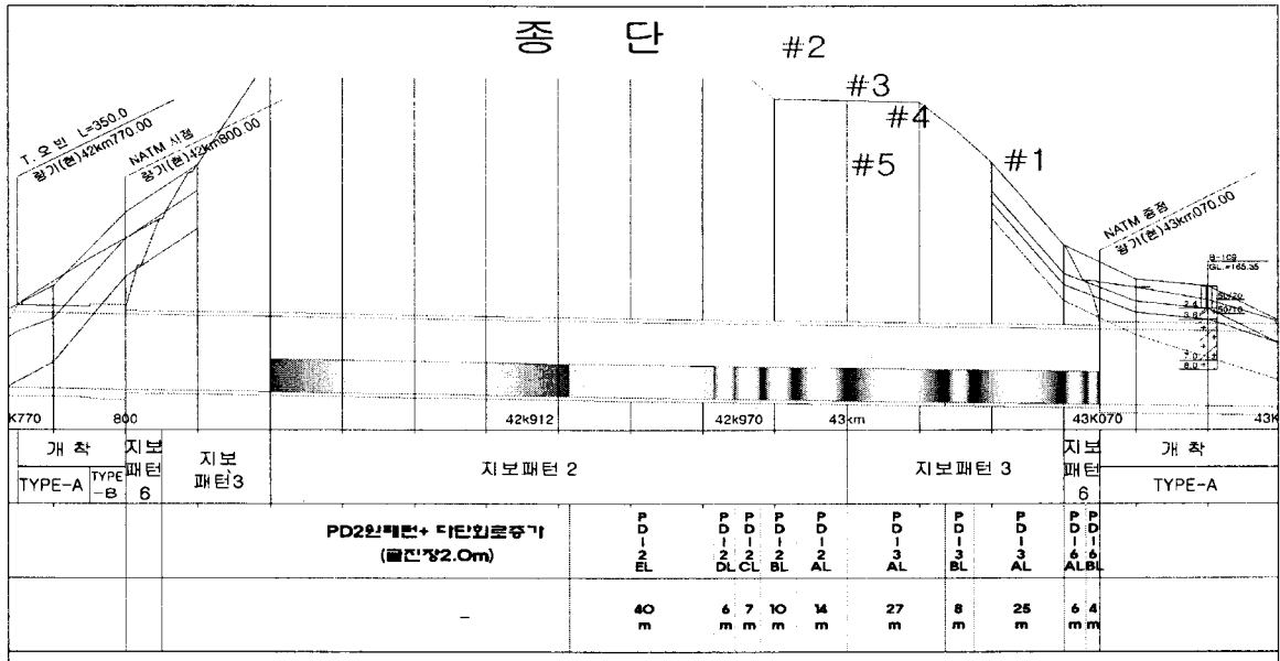
그림 3.1(b) 하단부터널 발파구간별 적용발파패턴 구분(단면도)
