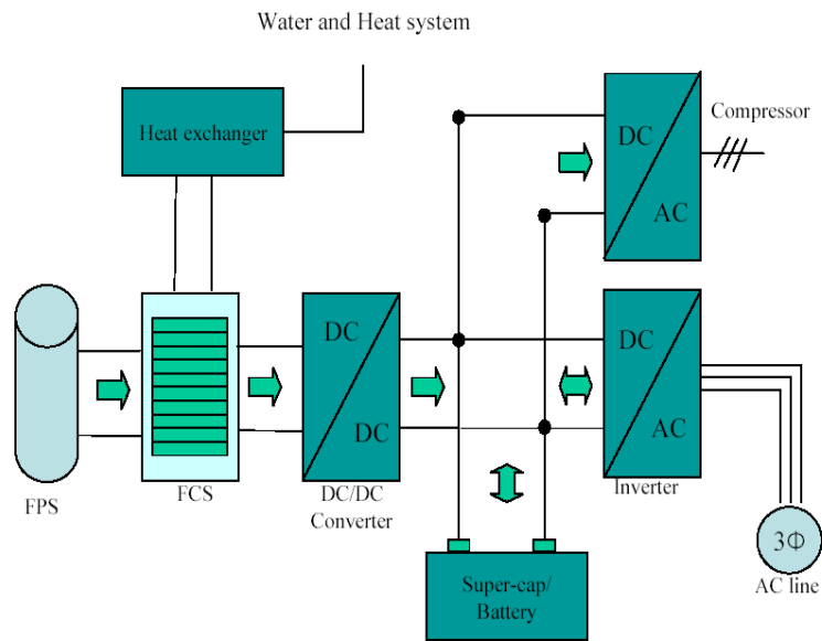
<그림 1> PEM fuel cell 전력변환장치 시스템의 구조
