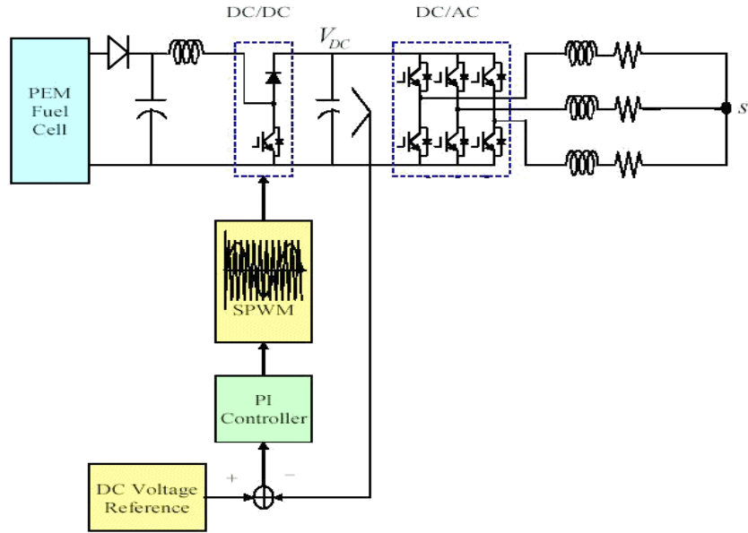
<그림 2> fuel cell 전력시스템
