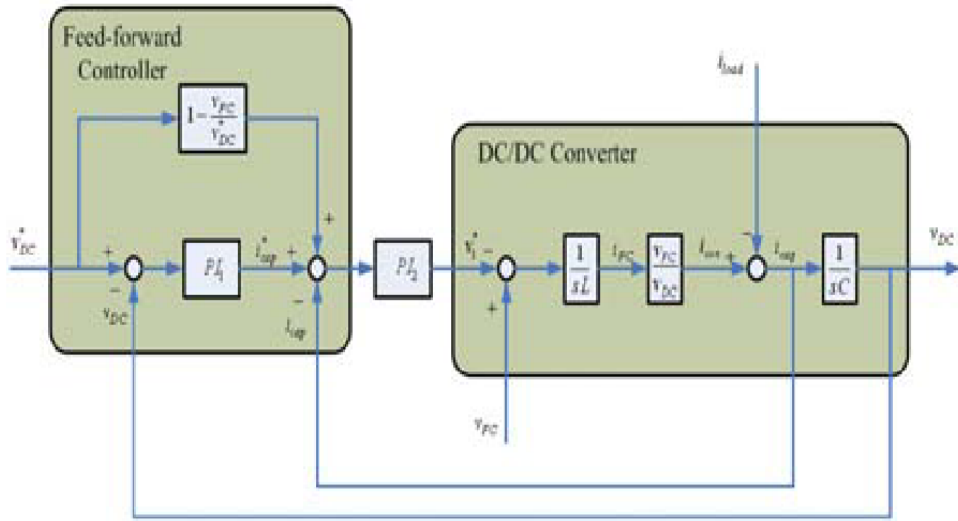
<그림 3> DC/DC converter 제어 블록 다이어그램
