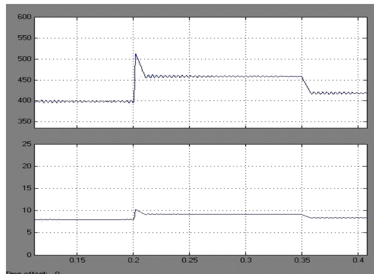
<그림 5> DC/DC converter 출력 전압/전류
