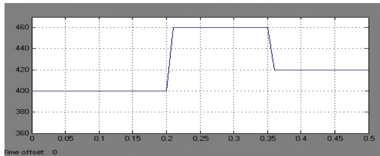
<그림 4> PEM fuel cell의 출력 전압 (DC/DC converter 입력 전압)
