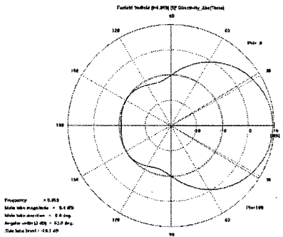
그림 10. H-평면 방사패턴 Fig 10. The Radiation Pattern of H-plane
