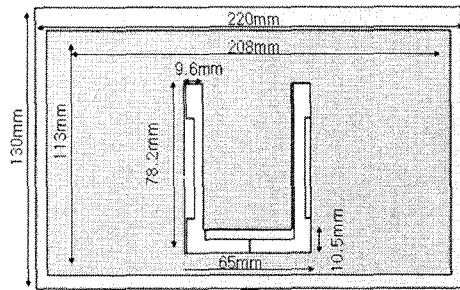
그림 7. U-Slot 안테나 전면 Fig 7. A Front of the U-Slot Antenna
