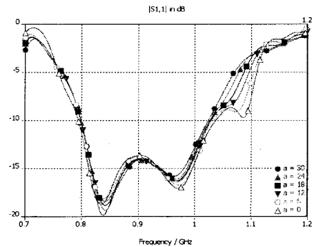
그림 2. (a)에 따른 S11의 변화 Fig 2. The Variation of S11 in terms of (a)
