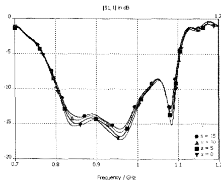
그림 6. (S)에 따른 S11의 변화 Fig 6. The Variation of S11 in terms of (S)
