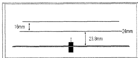
그림 8. U-Slot 안테나 측면 Fig 8. A Side of the U-Slot Antenna
