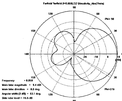
그림 11. E-평면 방사패턴 Fig 11. The Radiation Pattern of E-plane
