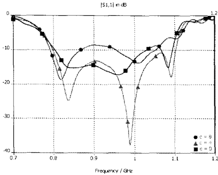
그림 5. (C)에 따른 S11의 변화 Fig 5. The Variation of S11 in terms of (C)
