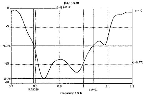
그림 9. 시뮬레이션 반사손실 Fig 9. The Simulated Return-loss
