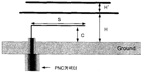
그림 4. 안테나의 구조 Fig 4. Structure of Antenna
