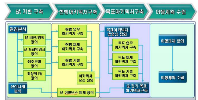
그림 10. 현행·목표 아키텍처 구축 절차
