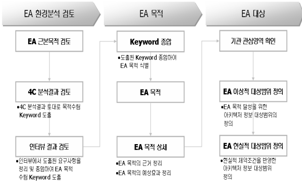
그림 7. EA 목적 및 범위 정의 절차
