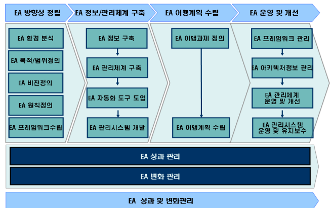
그림 5. 국방 EA 구축 절차
