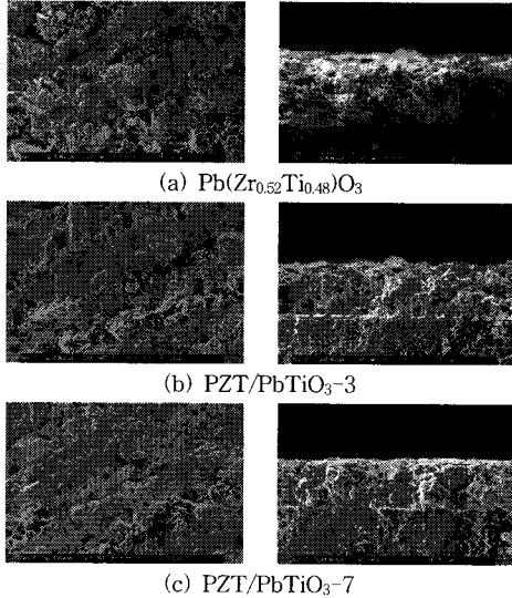
그림 2. PZT/PT 다층 후막/박막의 미세구조
