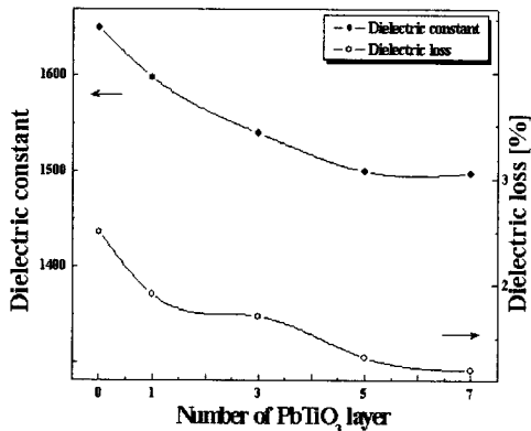
그림 3. PbTiO 3 코팅횟수에 따른 PZT/PT 다층 후막/박막/후막의 유전상수 및 유전손실
