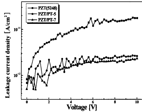
그림 4. PZT/PT 후막/박막의 인가전압에 따른 누설전류 밀도
