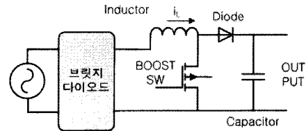
그림 3. 역률 보정회로
