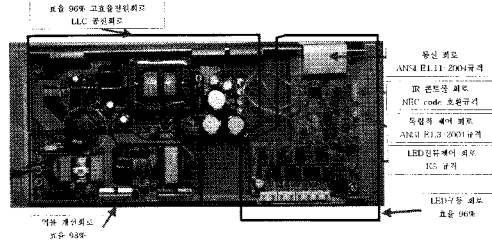
그림 4. 시제품의 외형
