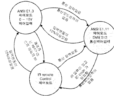
그림 3. 사용자 입력에 따른 조명단말기의 제어
