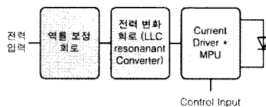
그림 2. 고효율 LED 구동회로의 구성
