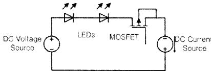
그림 7. LED 전류제어회로의 구성
