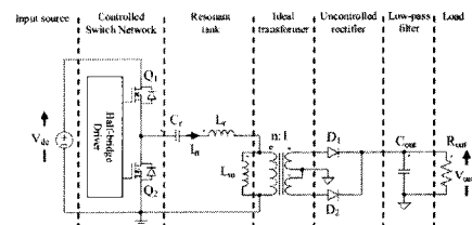
그림 5. LLC resonant Converter
