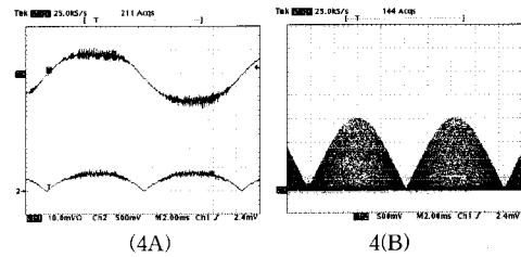
그림 4. 각단의 입력 전류와 출력 전류 4(a) 교류입력 전류와 다이오드 전류 4(b) MOSFET전류
