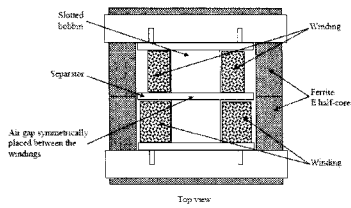
그림 6. LLC resonant Inductor -transformer
