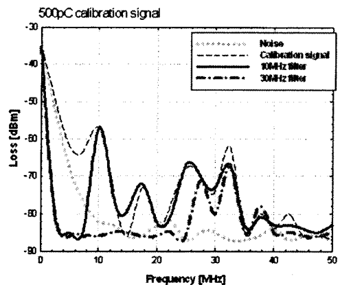
(a) 필터 적용 비교
