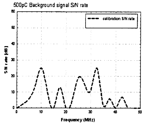
(b) calibration 신호의 S/N비
