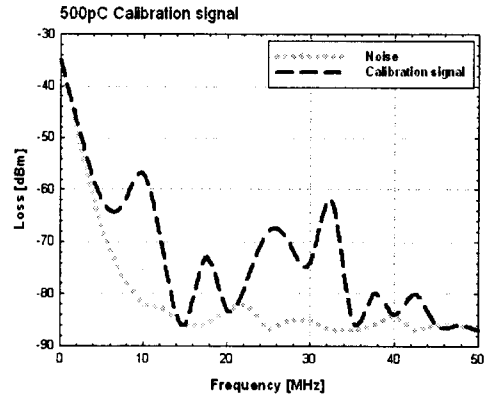
(a) Noise와 박전극 calibration 주입 신호 비교
