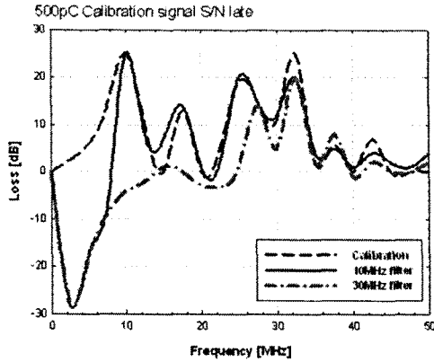
<그림 4> 필터 적용 후 NJB에서 주입된 calibration 신호
