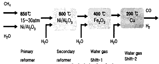
Fig. 1 개질반응의 과정
