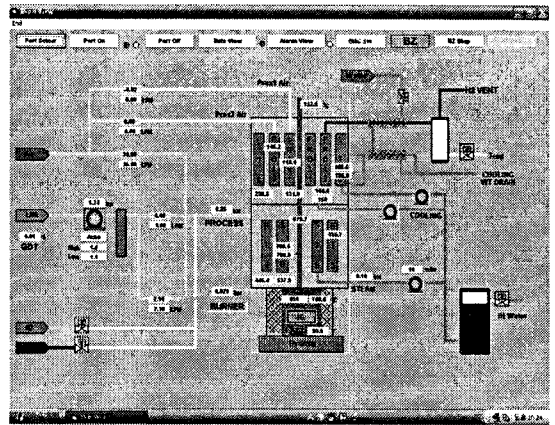
Fig. 3 운전중 모니터링 화면
