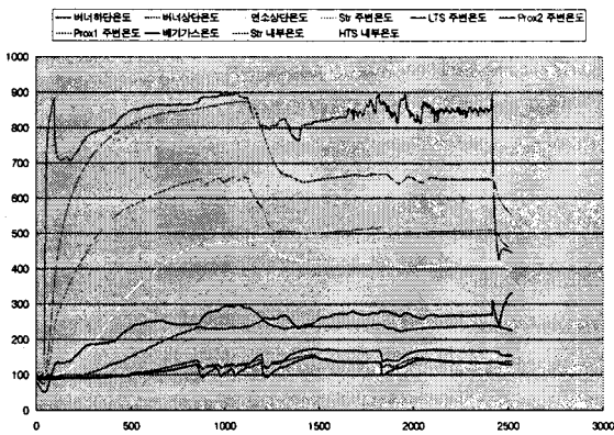
Fig. 5 구동시간에 따른 부분별 온도 특성
