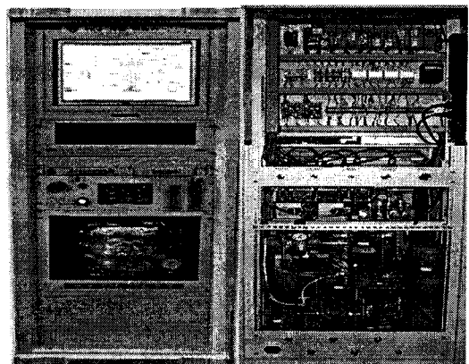
Fig. 2 동신대학교 개질 시스템
