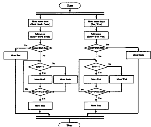
그림 2. 광센서 추적방식 제어 알고리즘.
