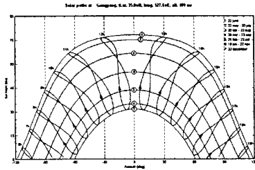
그림 4. 태양의 방위각 및 고도 변화.
