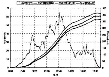
그림 9. 제어방식에 따른 발전량 비교.(제안한 방법)
