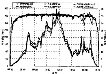
그림 8. 기후환경에 따른 직류전압 및 전류 비교.(제안한 방법)
