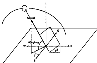
그림 3. 태양의 방위각 및 고도.
