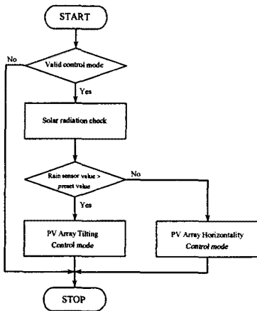
그림 6. 레인센서 변화에 따른 제어 순서도
