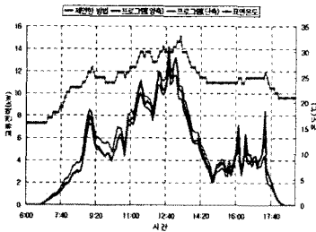
그림 7. 기후환경에 따른 표면온도 및 교류전력 변화.(제안한 방법)
