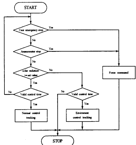
그림 5. 일사량 변화에 따른 제어 순서도.
