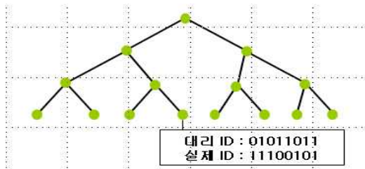
<그림 4 : 난수 트리 위킹 알고리즘>
