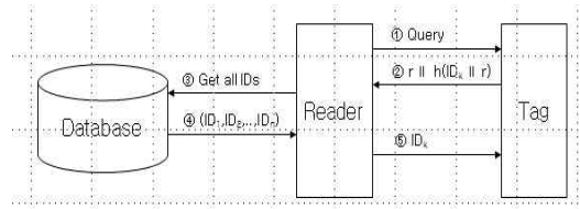
< 그림 2 : Randomized Hash-Lock >
