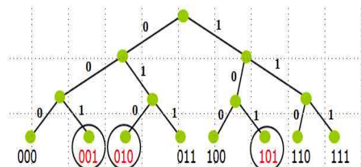
<그림 3 : 트리 워킹 알고리즘 >
