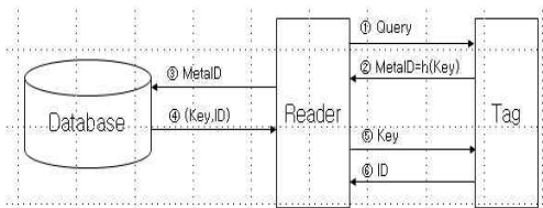
<그림 1 : Hash Lock >
