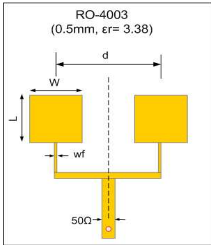
그림 2. 실제 제작된 안테나 모양 (W=4.2mm, L=3.2mm, wf=0.1mm, d=6mm)
