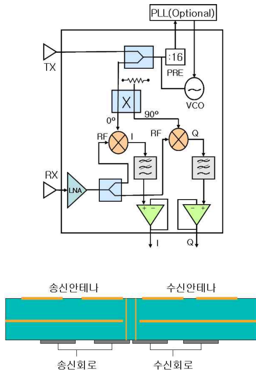
그림 1. 차량충돌 방지용 송수신기 회로 및 안테나 배치도
