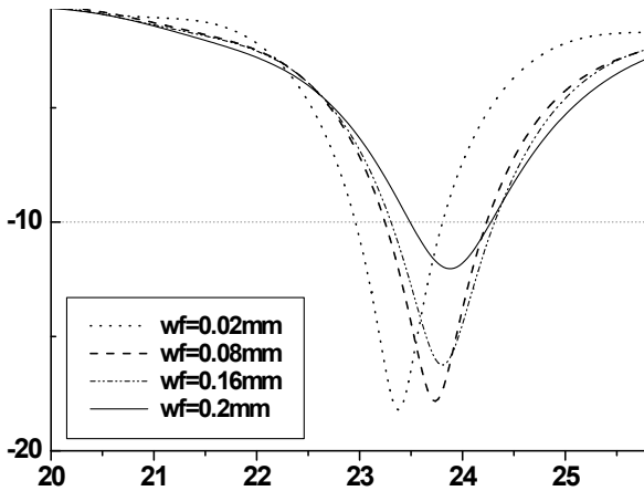
그림 3. 안테나 시뮬레이션 결과
