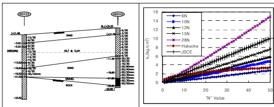
Fig. 5. 지반조건 및 수평지반반력계수
