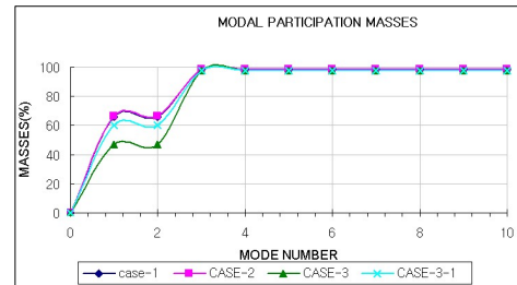
Fig. 7. 해석별 질량참여율
