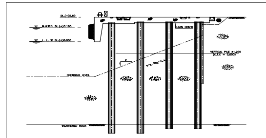
Fig. 2. 잔교식 안벽의 해석단면
