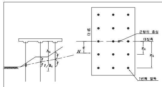
Fig. 1. 가상지표면의 산정방법
