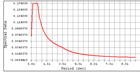
Fig. 6. 표준설계응답스펙트럼
