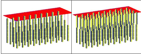
Fig. 4. 지반스프링 해석모델링
