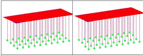
Fig. 3. 고정단 해석모델링
