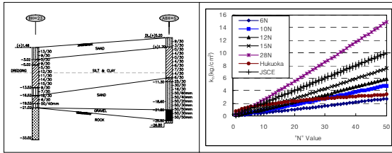
그림5. 지반조건 및 수평지반반력계수
