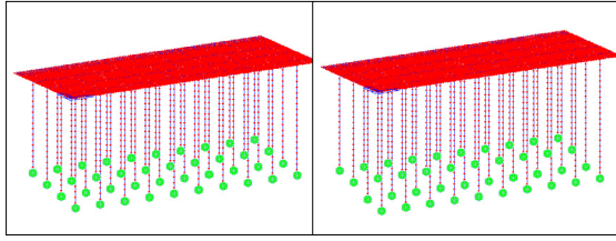
그림3. 고정단 해석모델링
