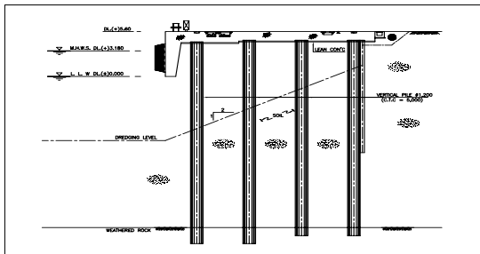
그림2. 잔교식 안벽의 해석단면
