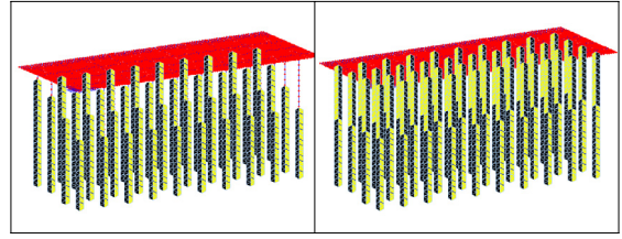
그림4. 지반스프링 해석모델링
