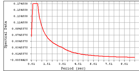
그림6. 표준설계응답스펙트럼
