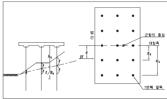
그림1. 가상지표면의 산정방법
