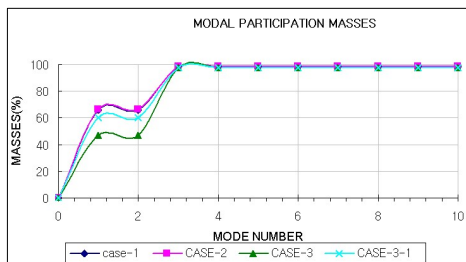
그림7. 해석별 질량참여율
