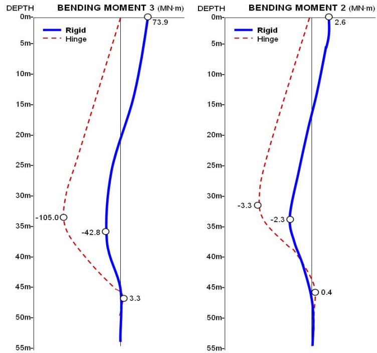
그림 15. 말뚝머리 구속 조건에 따른 깊이별 휨모멘트 분포
