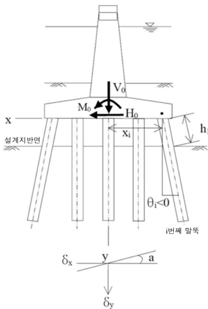
그림 5. 탄성변위법의 계산좌표
