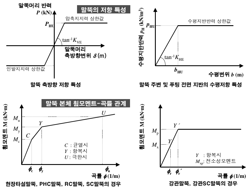
그림 9. 말뚝의 저항특성, 휨모멘트와 곡률 관계 (日本道路協會, 2002)
