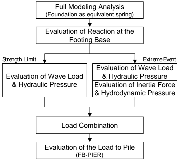
그림 13. 말뚝 하중 산정 절차
