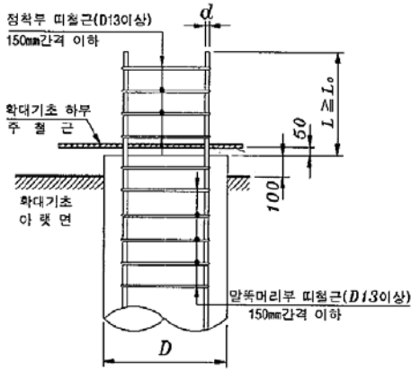
그림 3. 현장타설말뚝 강결합 방법-B의 구조세부
