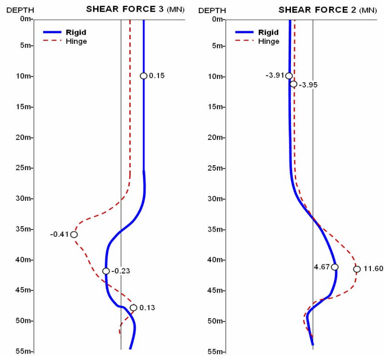
그림 16. 말뚝머리 구속 조건에 따른 깊이별 전단력 분포
