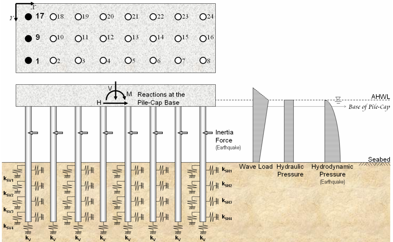
그림 12. 다주식 기초 구조계에 작용하는 외력과 기초의 모델링
