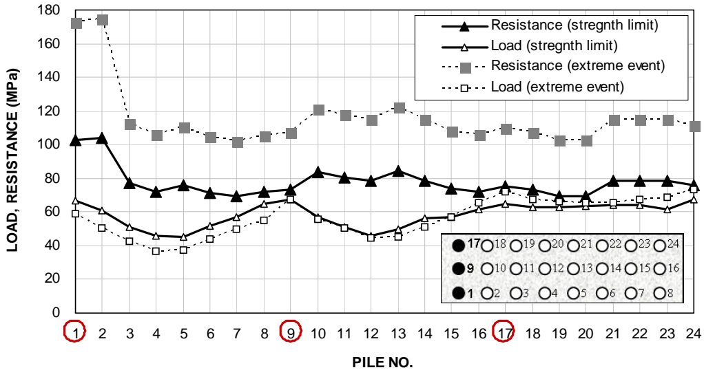
그림 21. 파일캡 하단 24개 말뚝의 연직하중과 연직지지력 비교
