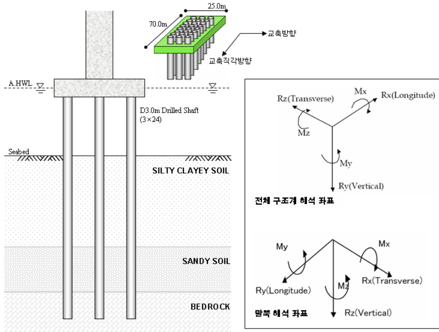
그림 10. 해석 대상 구조물 모식도 및 구조계별 해석 좌표
