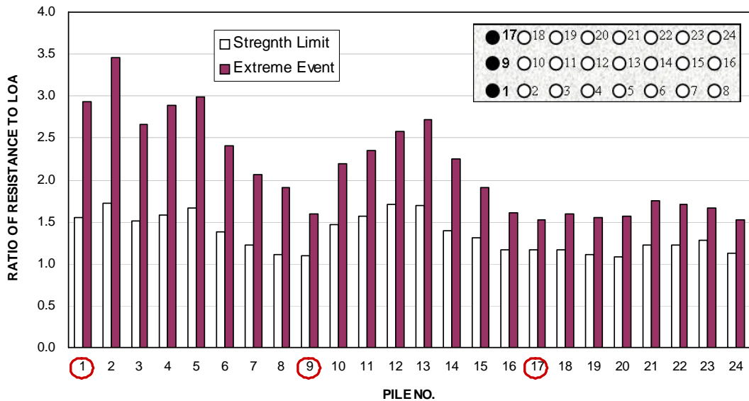
그림 22. 파일캡 하단 24개 말뚝의 하중/지지력 비 비교 (평상시 및 지진시)
