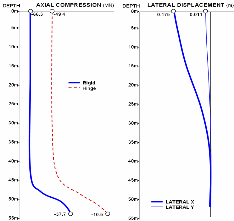
(a) 구속조건별 축방향 압축력 (b) 강결합 조건의 횡변위 그림 17. 말뚝 길이별 축력과 횡변위 분포
