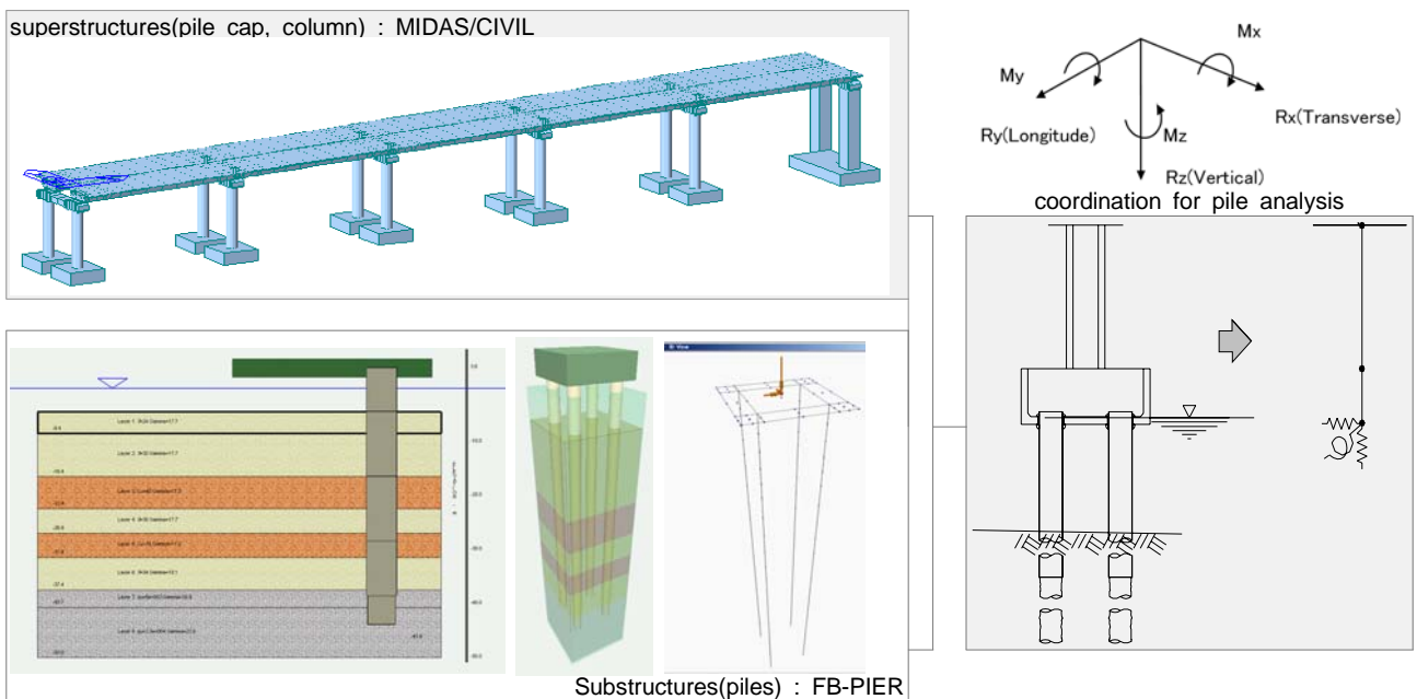
그림 11. 파일캡 기초 형식의 구조해석 모델링 개념
