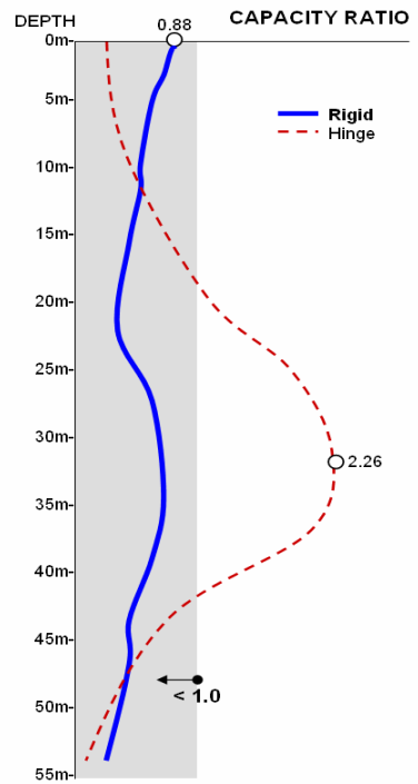
그림 18. 말뚝머리 구속 조건에 따른 부재 검토 결과
