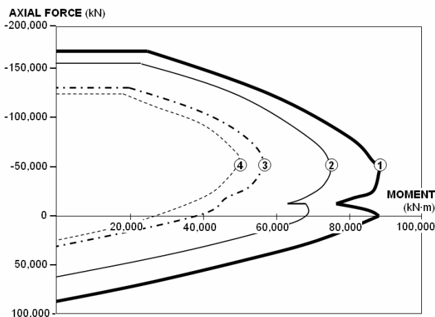
그림 19. 말뚝의 축방향 강성 변화에 따른 단면의 PM 상관도
