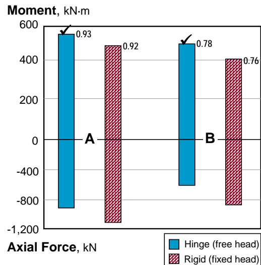
그림 6. 파일캡이 지중에 설치되는 강관말뚝 기초에서 말뚝머리 구속 조건에 따른 축력과 모멘트 비교
