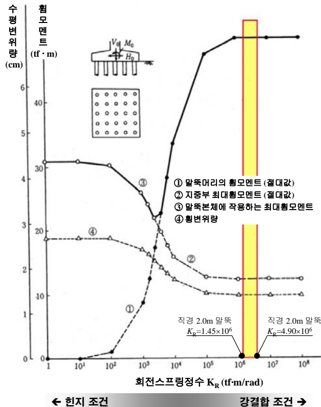
그림 7. 말뚝머리 연결 조건과 회전스프링정수의 관계 분석
